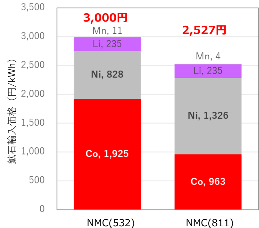
1kWhのLIBに必要な原料鉱石の輸入価格
