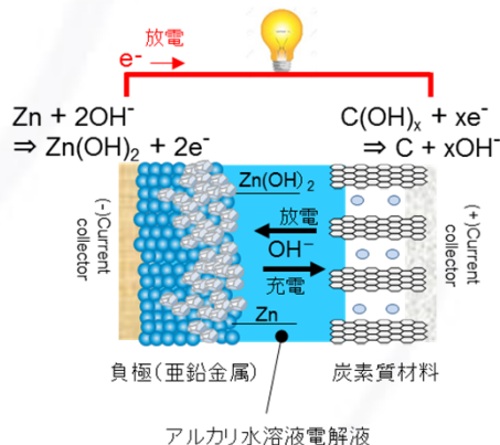
亜鉛負極電池
