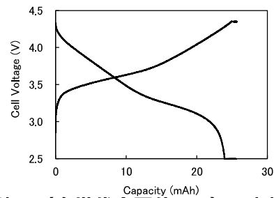
実証セル（次世代全固体LIB）の充放電曲線
