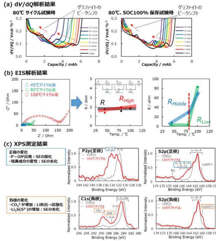
全固体LIBの劣化解析結果
