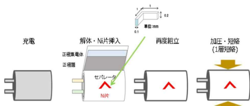
IEC62660-3の強制内部短絡試験の方法
