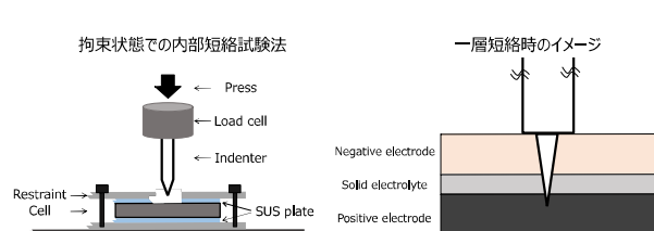
開発した全固体LIBの強制内部短絡試験法 （Niネイル短絡試験）の概要
