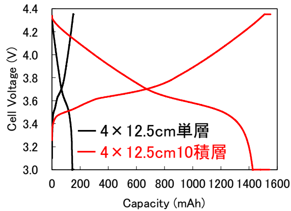
図 3.1.1-4 積層実証セル(第 1 世代全固体 LIB)の充放電曲線
