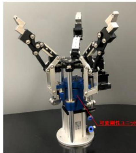
試作した可変剛性機構搭載の試作ロボットハンド (フレキシブルな把持と堅牢性を兼ね備える。)
