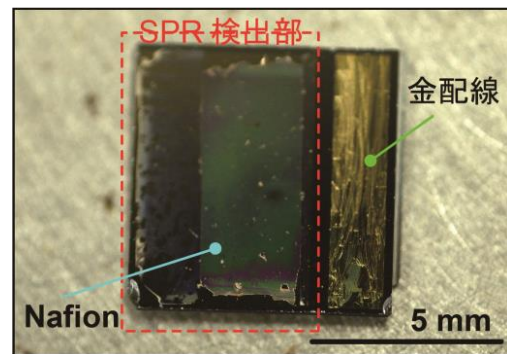
Si-SPR センサ上にナフィオン膜を塗布したセンサの試作デバイス
