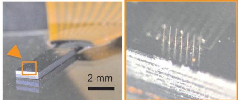
作製した多チャンネルシリコンプローブ電極デバイス
