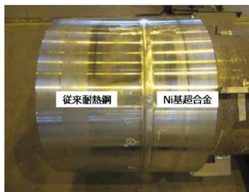
ロータ異材溶接部(例)
