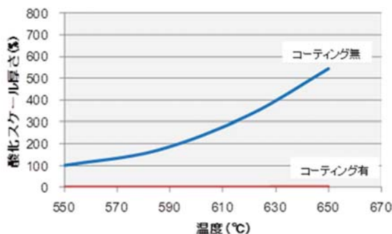
高Cr鋼の酸化スケール生成厚さ(例)
