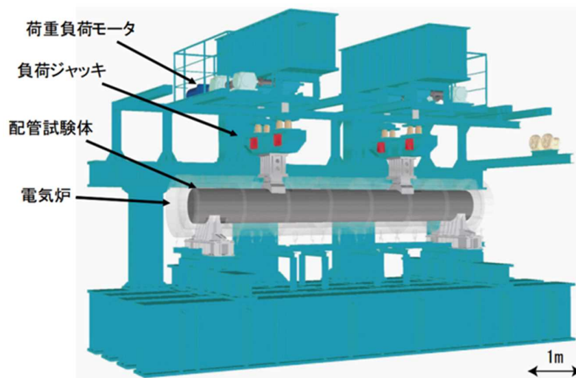
図 3-1 大径管内圧クリープ試験装置（BIPress）
