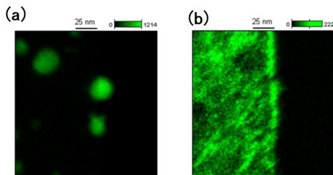
図 III.2.1.1.3.1-3 化合物 N4 表面に担持された助触媒 B の TEM-EDS (エネルギー分散型 X 線分光法) によるマッピング像 (a) 含浸法により担持、(b) 新手法により担持
