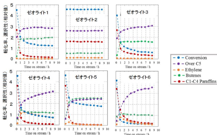
図Ⅲ.2.2.5.2.2-1 各種ゼオライトにおけるプロピレン転換反応結果
