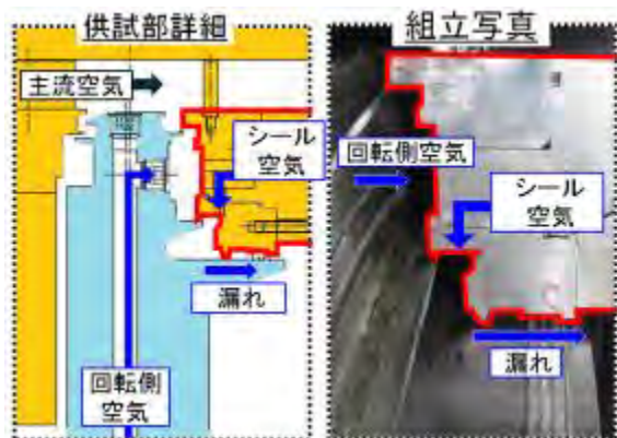
図④-a1 シール試験装置
