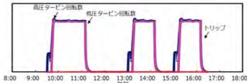
図 2017/10/13の運転データ
