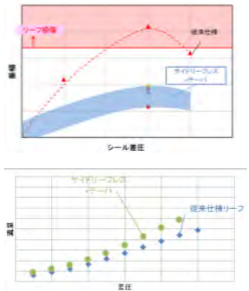
図⑧-2 要素試験結果
