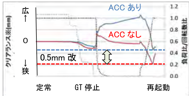
図⑦-3. クリアランス履歴
