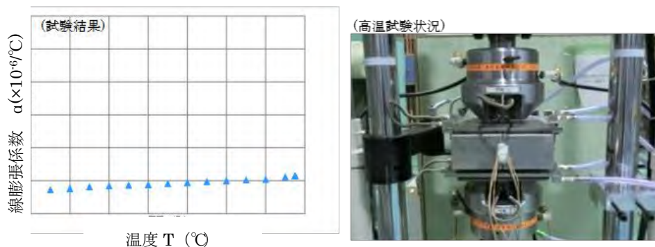
図②-2 高耐熱性材料を用いた熱構造設計向け 基礎データ
