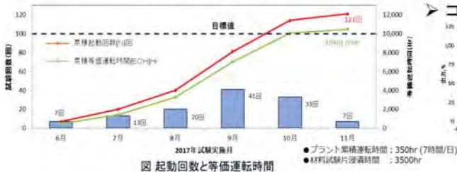
図 起動回数と等価運転時間
