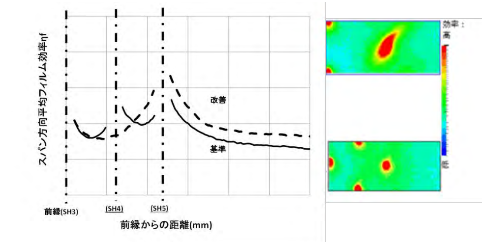
図②-1 シャワーヘッド冷却部冷却性能 計測結果
