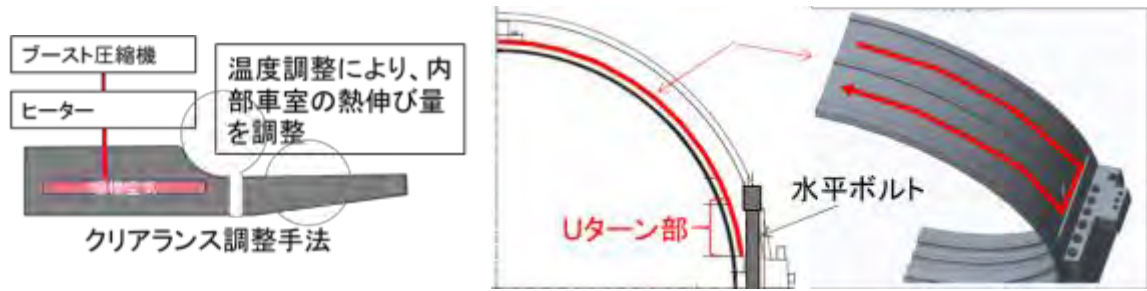
図⑦-1. クリアランスコントロール構造
