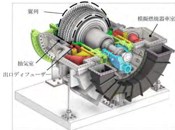
図⑥-3 後方段模擬試験装置
