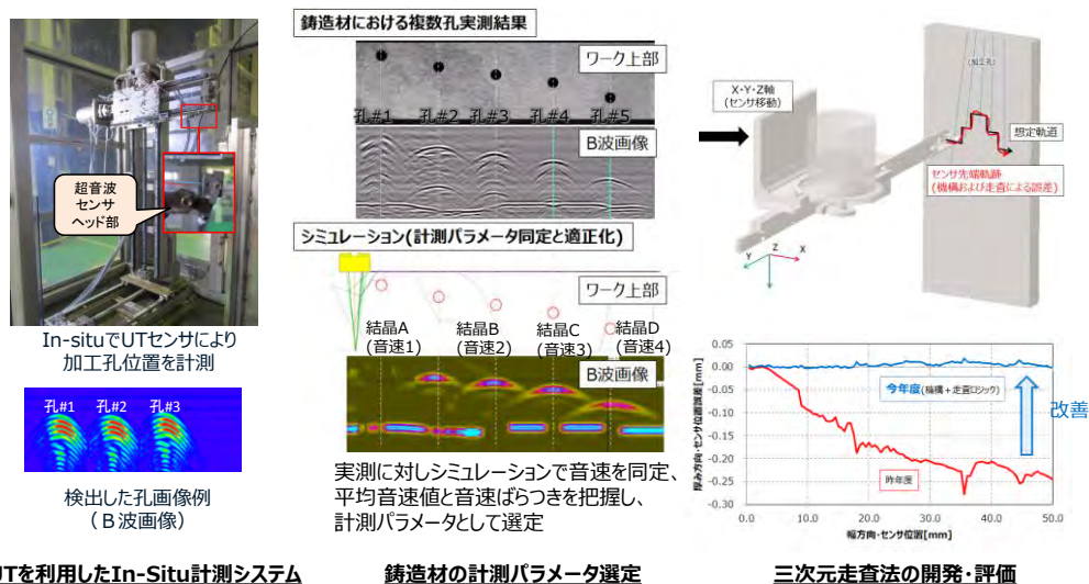
図⑨-3 複数孔同時計測システムの開発
