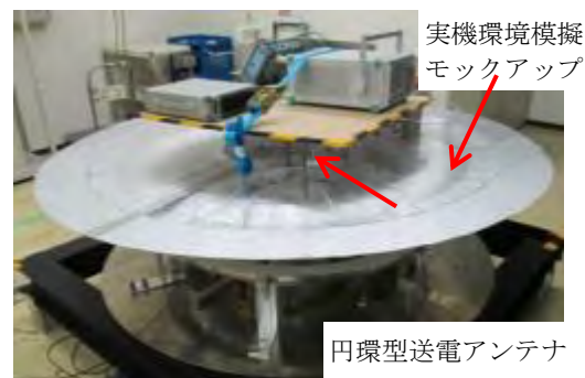
図⑬-（2）-2 実機環境下検証システム
