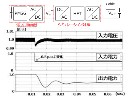
図3-39 DC-DC変換器のシミュレーション検討
