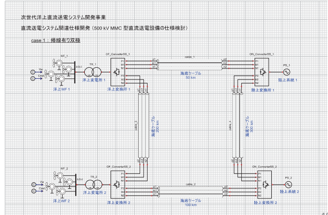
図3-13 XTAPで作成した双極ケース(帰線有)
