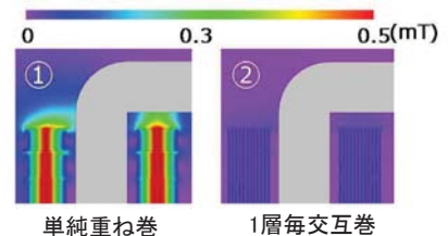
図3-38 漏れ磁束の計算結果(コンター図)
