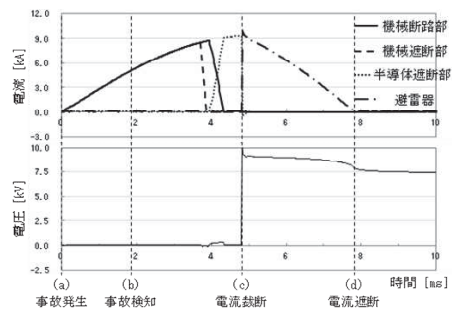
図3-19 遮断試験結果波形
