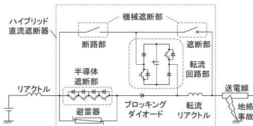
図3-1 ハイブリッド直流遮断器の構成
