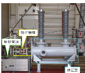
図3-14 断路部性能検証
