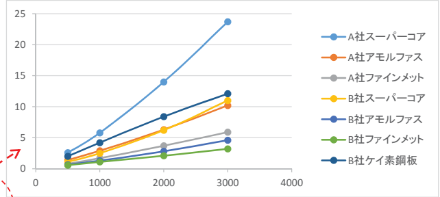
図3-32 コア材料の周波数特性
