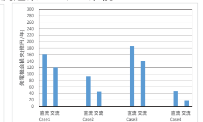
図3-8 発電機会損失の比較(暫定)
