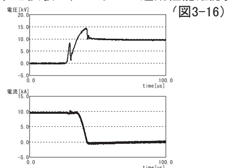
図3-16 半導体遮断部遮断波形
