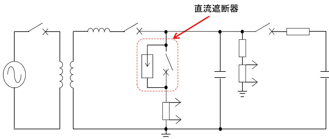
図 3-4-6 試験回路
