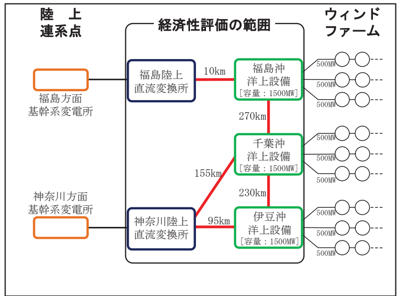
図3-3 経済性評価の範囲(直流連系)
