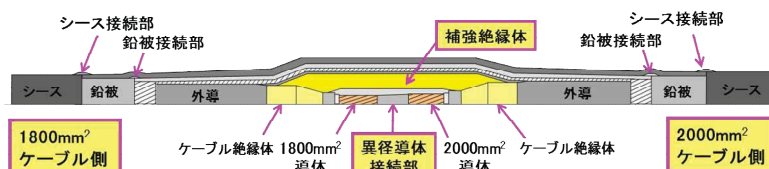
図3-23 異径ケーブルの工場接続部断面図
