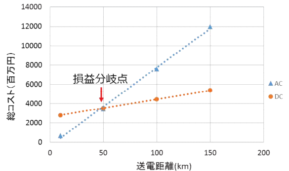
図3-9 年経費(総コスト)と送電距離の関係 40
