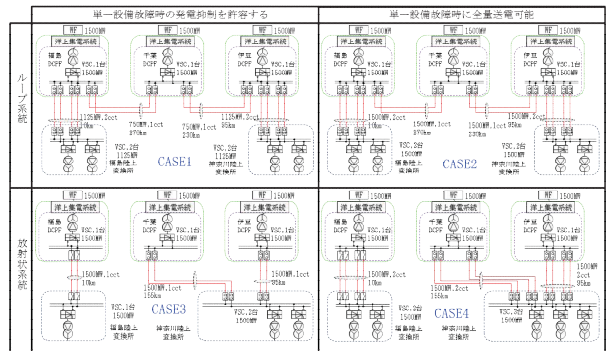
図3-5 直流連系のモデル系統
