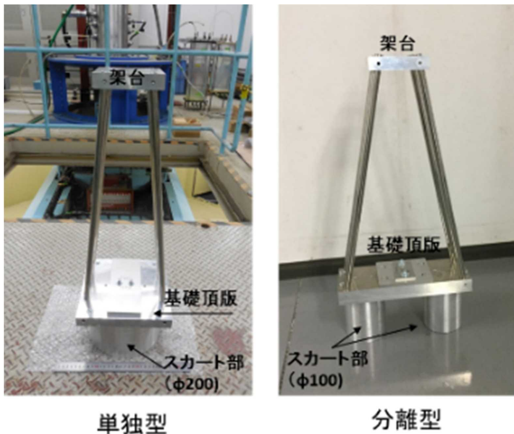
図 3-6-2 実験模型
