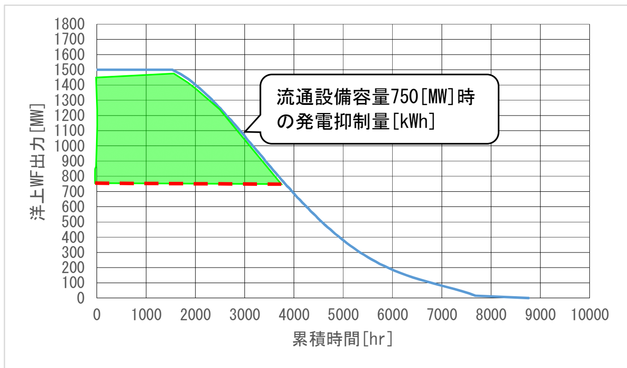
図 3-2-5 洋上 WF の出力-累積時間曲線と発電抑制量
