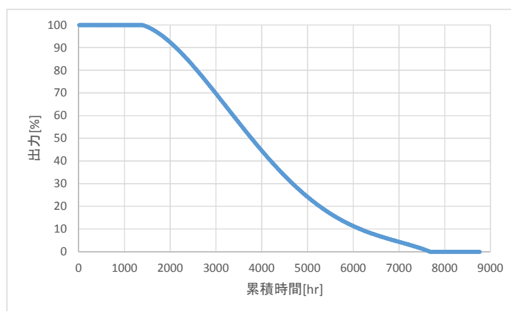
図 3-2-2 洋上 WF の想定出力-累積時間特性
