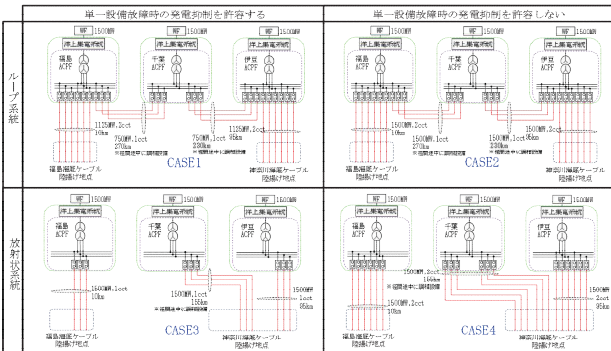
図3-4 交流連系のモデル系統
