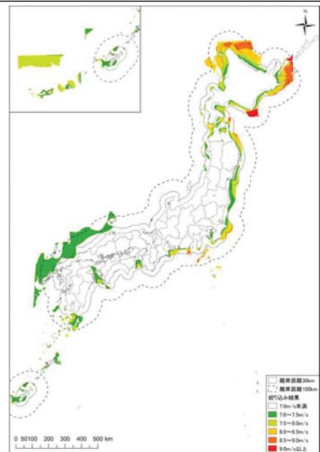
図3-1 ポテンシャルの高い地域の抽出結果
