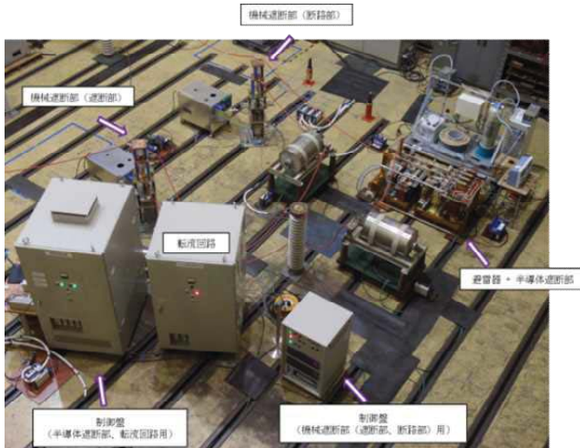
図3-17 ハイブリッド直流遮断器10kVモデル
