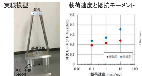
図3-27 遠心力模型実験結果
