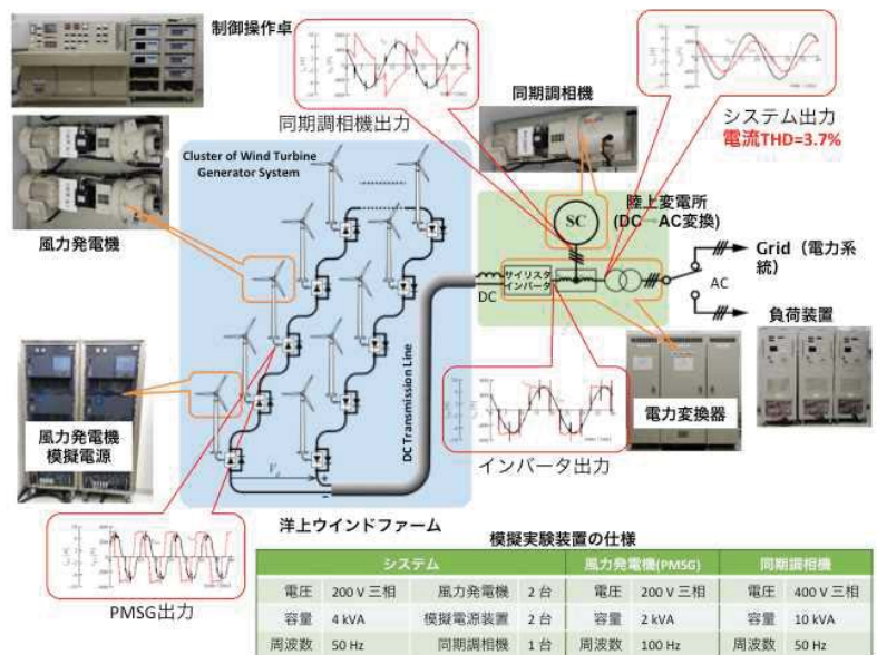
図3-30 直列接続方式風力発電システムの構成と模擬実験装置 (実験結果は系統連系運転出力2.7kW時の電流(Red),電圧(Black)の波形例)
