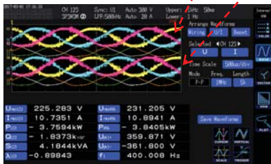
図3-34 高周波変圧器・実験結果
