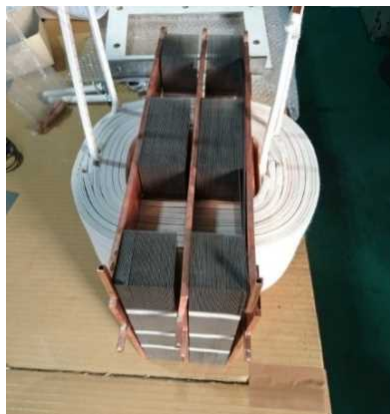
図 3-7-9 水冷高周波変圧器と熱流解析結果 (ポンプ動力 vs. 熱伝達率)
