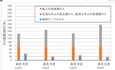
図3-7 送変電損失の比較(暫定)
