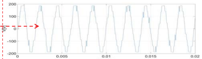
図3-33 リアルタイムシミュレータMMC変換器出力波形
