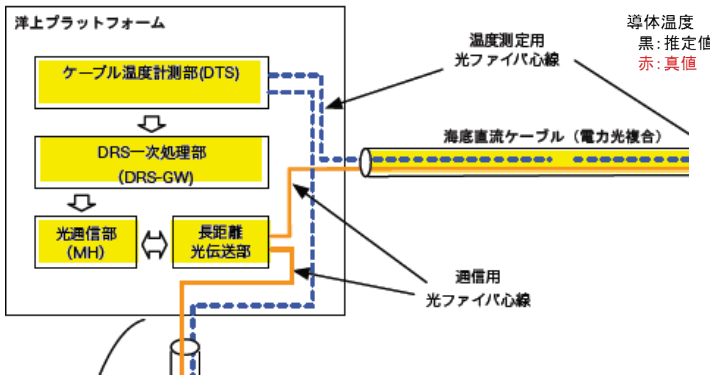
図3-20 プラットフォーム間のダイナミックレイティングシステム
