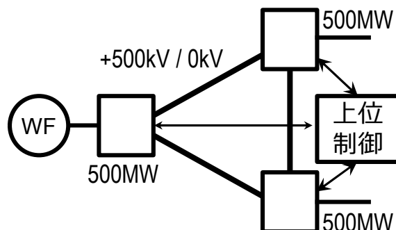
図 3-3-6 非対称単極 3 端子系統
