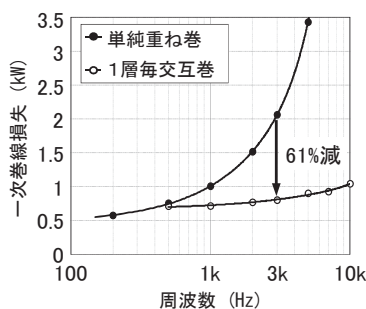
図3-37 1次巻線損失の周波数特性(500kVA)
