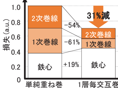
図3-40 全損失比較(500kVA)
