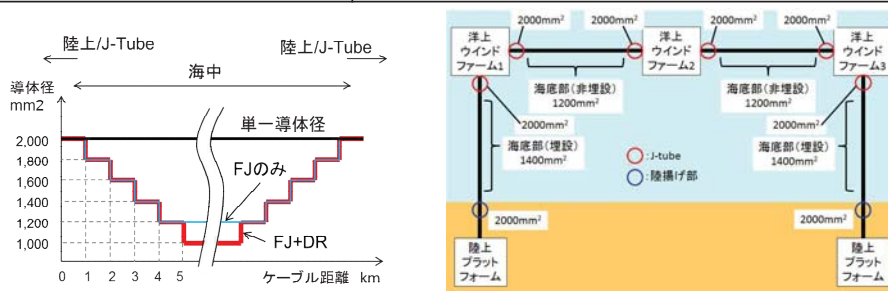
図3-22 異なる導体断面積のケーブルで構成する洋上直流送電システムの一部
