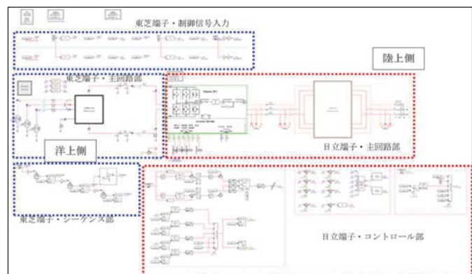
図3-12 単極2端子の組み合わせモデル(RTDS)
