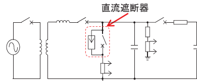
図3-18 試験回路
