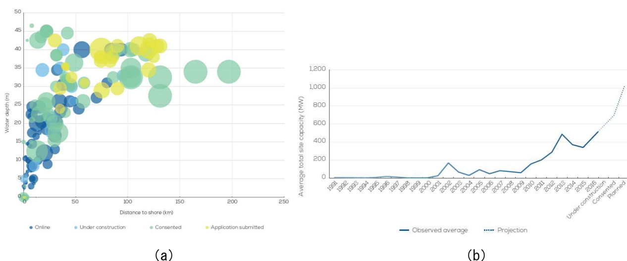
図1-5 欧州における洋上WFの規模と離岸距離と深さの推移（a）、洋上WF容量の推移（b）
