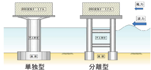
図3-26 洋上PFにサクシオン基礎を適用したイメージ図
