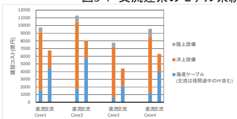
図3-6 設備経費の比較(暫定)
