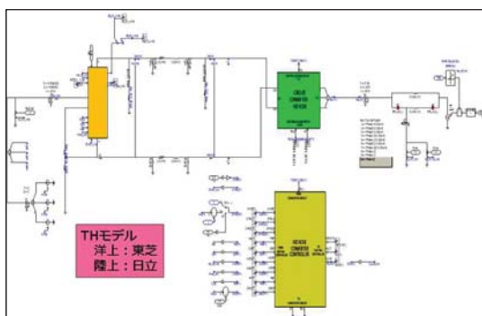
図3-11 単極2端子の組み合わせモデル(PSCAD)
