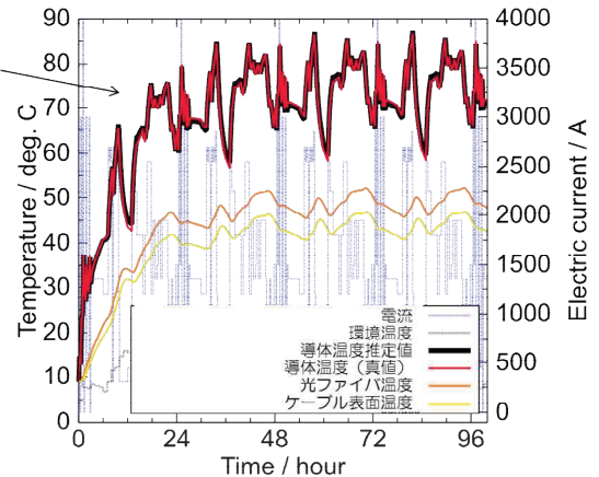
図3-21 開発した導体温度推定アルゴリズムの結果の一例
