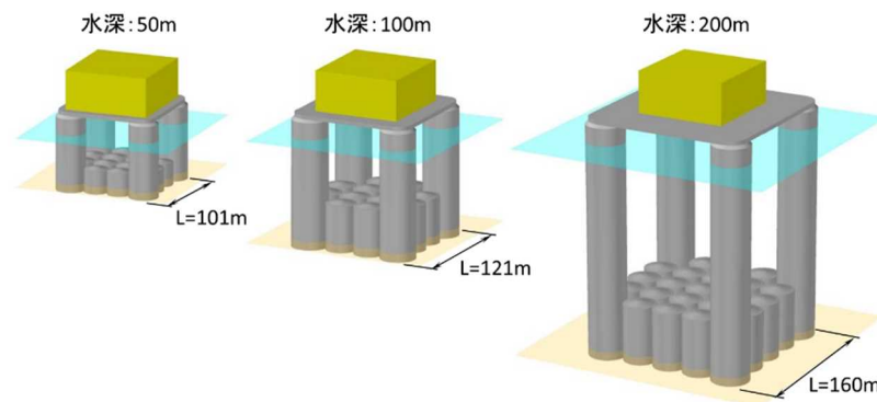
図 3-6-6 概略設計結果
