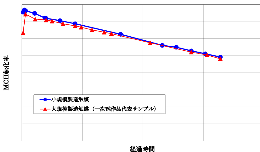
図 9 商業生産触媒ラボ評価例
