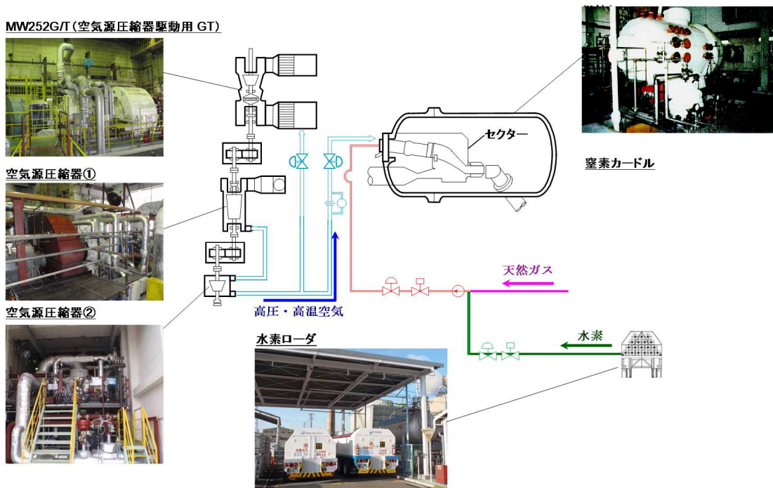
図 3.4 実圧燃焼試験設備系統概略図
