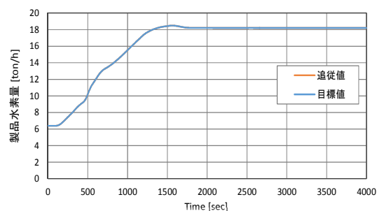
図 7 解析結果例 製品水素流量
