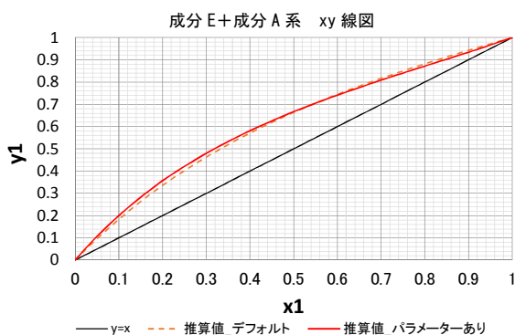
図3 蒸留シミュレーターへの気液平衡データ反映例
