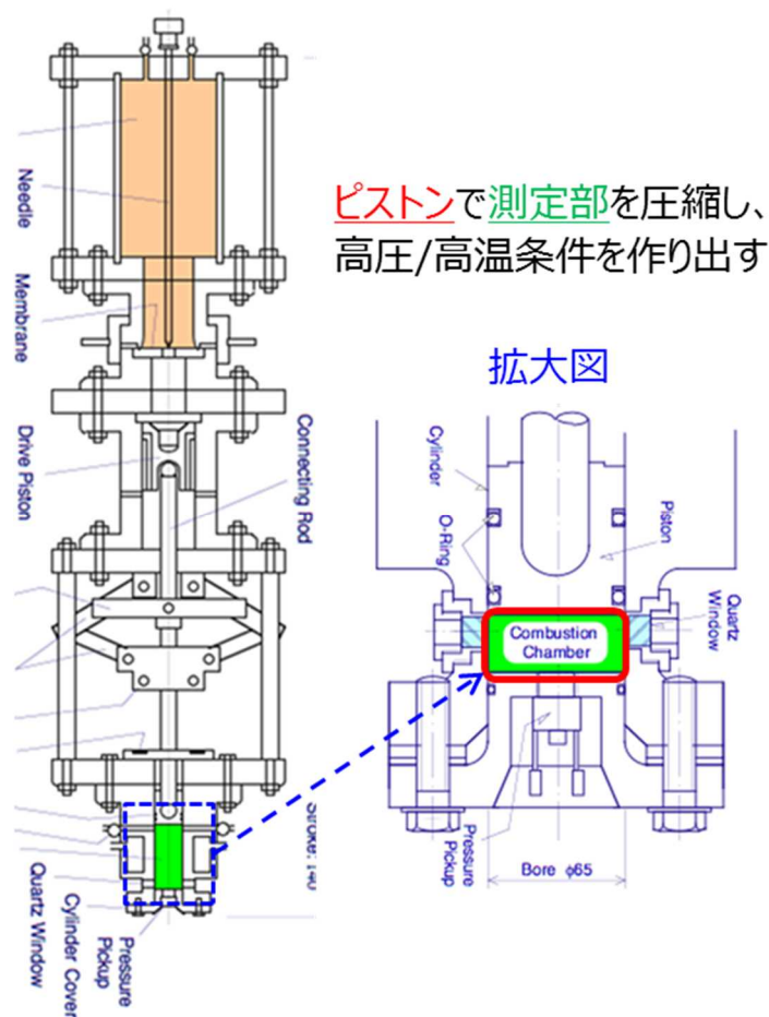
図 3.2 急速圧縮器
