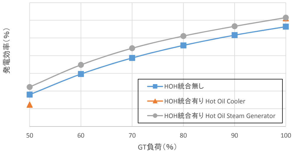
図 13 HOH の有無による発電効率比較
