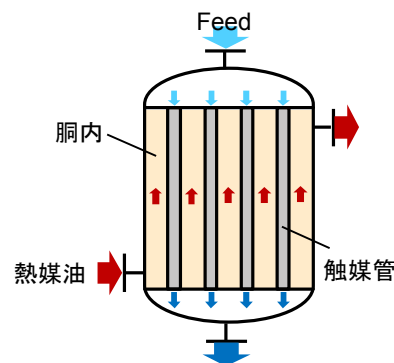
図5 脱水素反応器概念図
