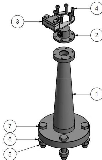
図 6 試験用レーダー式液面計
