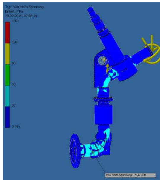
図 9 接続部構造解析
