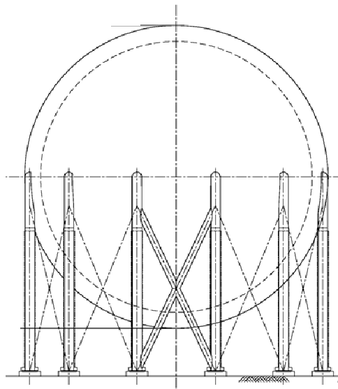
図 10 液化水素貯蔵タンク外形図
