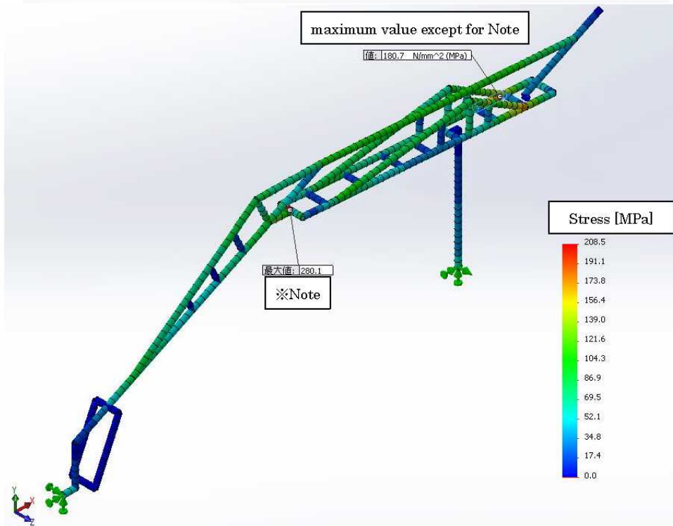
図 8 アーム部の各状態における構造解析
