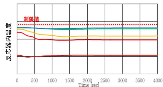
図 8 解析結果例 反応器内温度
