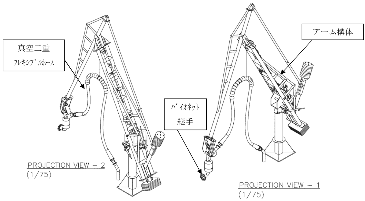
図7 ローディングシステム外形図
