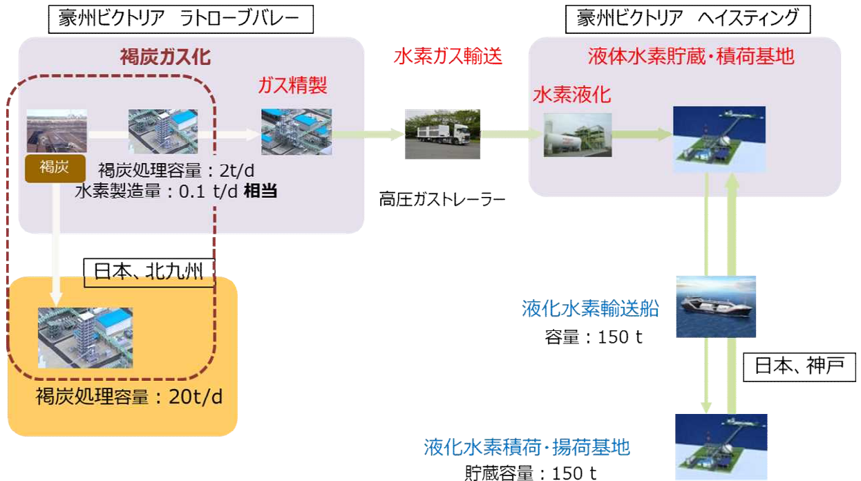
図 12 サプライチェーンにおける褐炭ガス化プロジェクトの概要
