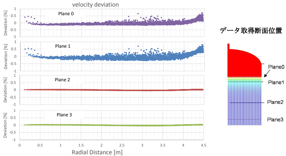
図6 定格ロード時の触媒管水平断面体積流量偏差
