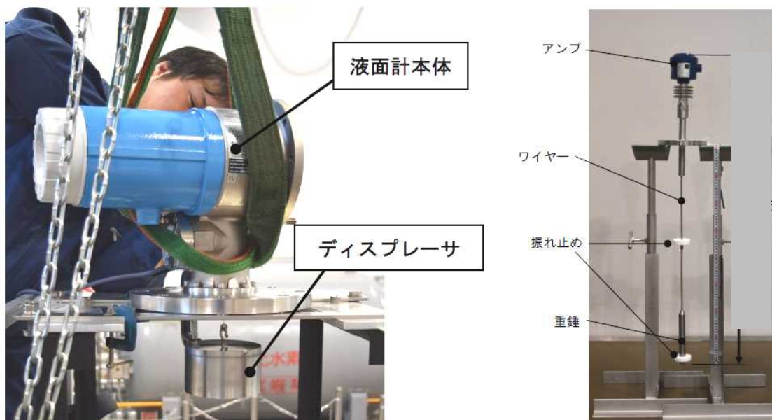
図 5 液面計試験装置 (左: ディスプレーサ式、右: 静電容量式)
