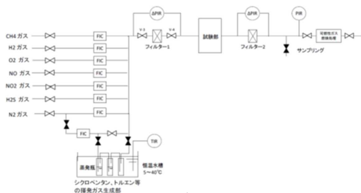
図 12 試験システム図
