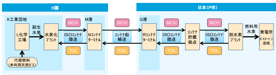
図 14 実証チェーン概略フロー
