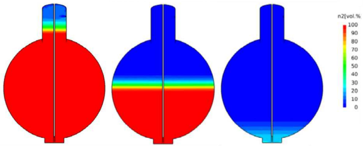
図 4 貨物タンクガス置換 数値解析モデル計算結果例
