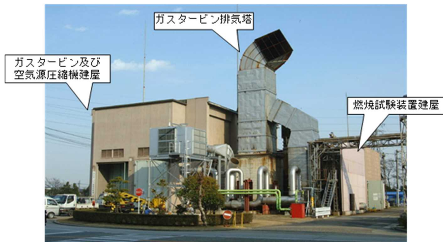
図 3.3 実圧燃焼試験設備外観
