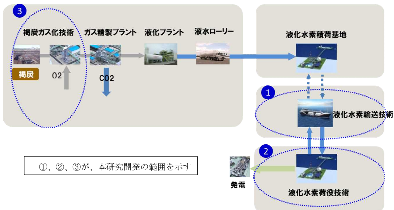
図 1 液化水素チェーンの概要
