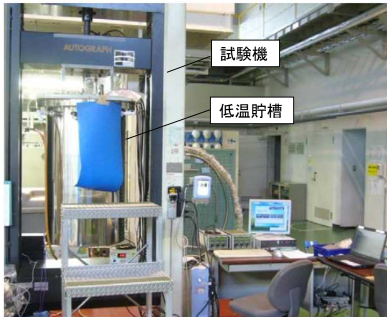
図 3 破壊靱性試験、試験状況
