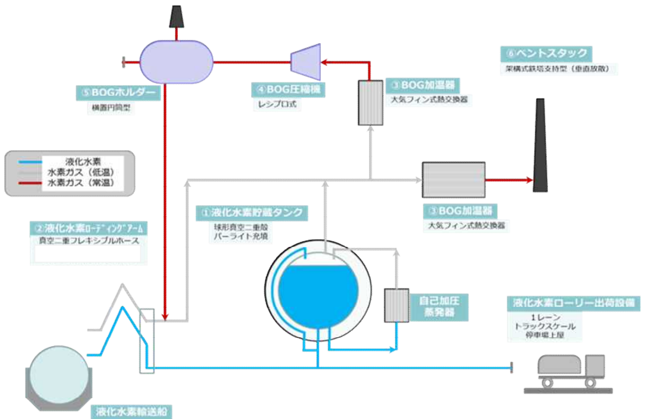
図 11 荷役基地 概略フロー
