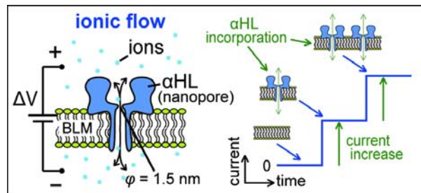
図 -(1A)-1.4 ヘモリシン (HL) による膜貫通孔の電気特性
