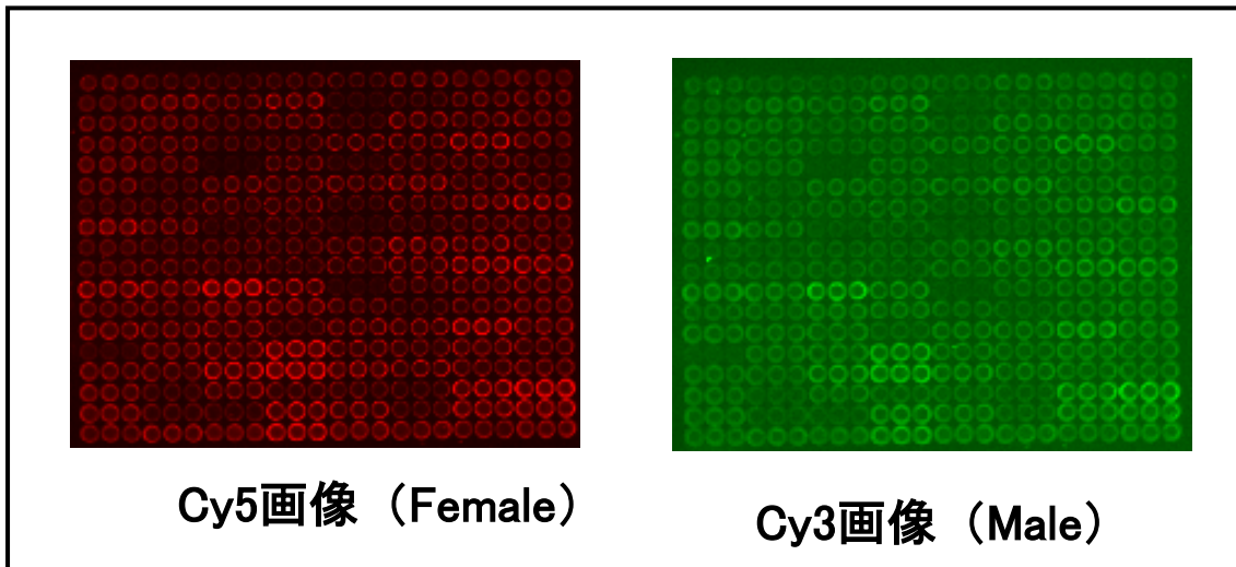
図 2.3-③-2 144 ミニアレイのハイブリ結果
