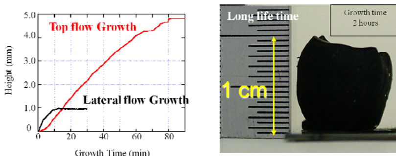
図 III-23 シャワーヘッドで成長の長寿命化と高さ1センチのSGCNT成長に成功
