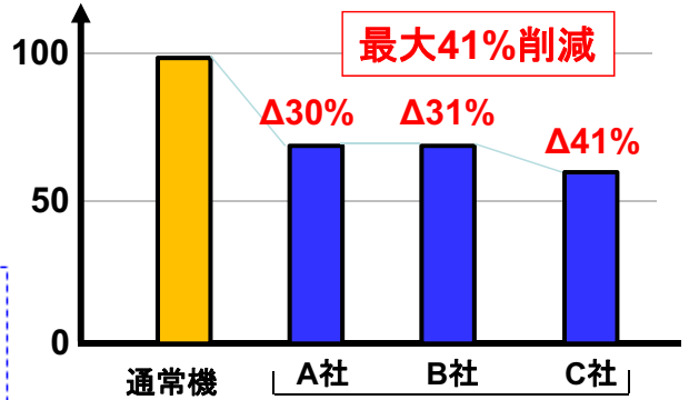
PC200-8ハイブリッドの燃料消費量(通常機比)
