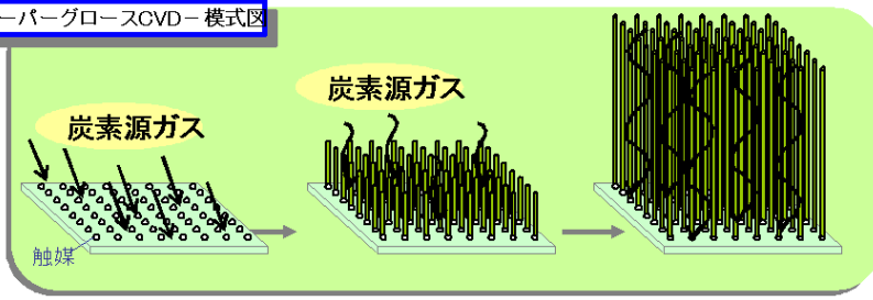
スーパーグロースCVD-模式図
