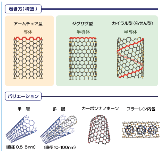
CNTの分類 (出典: NEDOホームページ)
