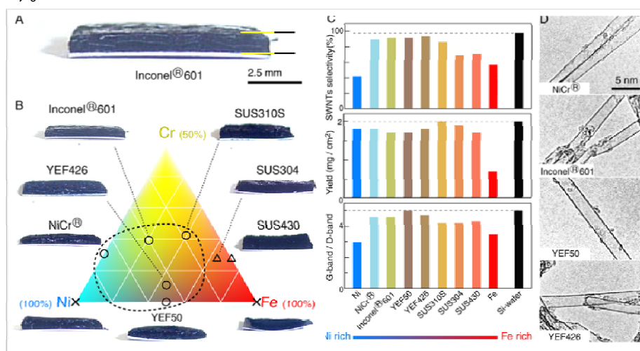
図 III-20 ニッケル合金基板上での SGCNT 合成
