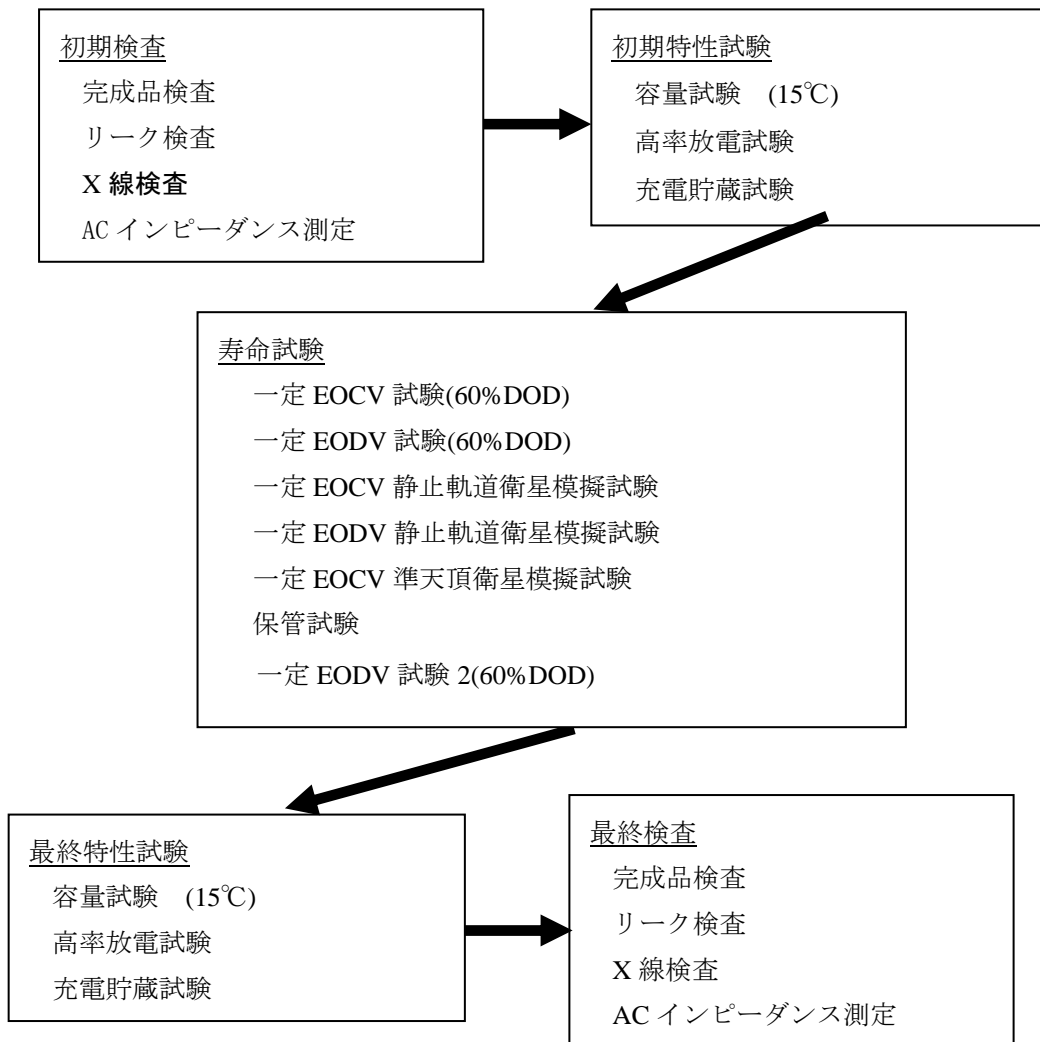
図 3.2.12.1-1 寿命評価試験フロー
