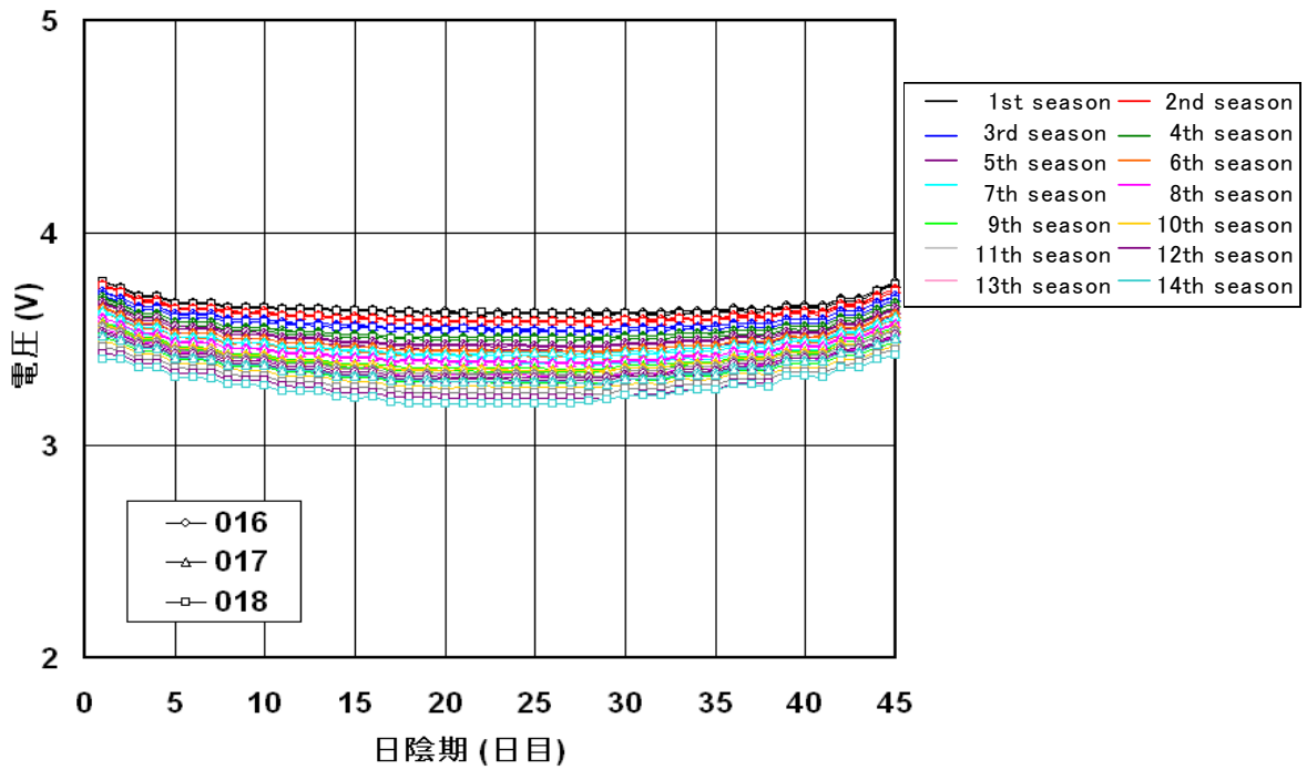
図 3. 2. 12. 2-7 一定 EOCV 静止軌道模擬試験の EODV 推移.
