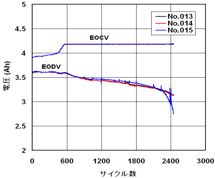
図 3.2.12.2-3 一定 EODV 試験 1 中の EOCV と EODV の推移
