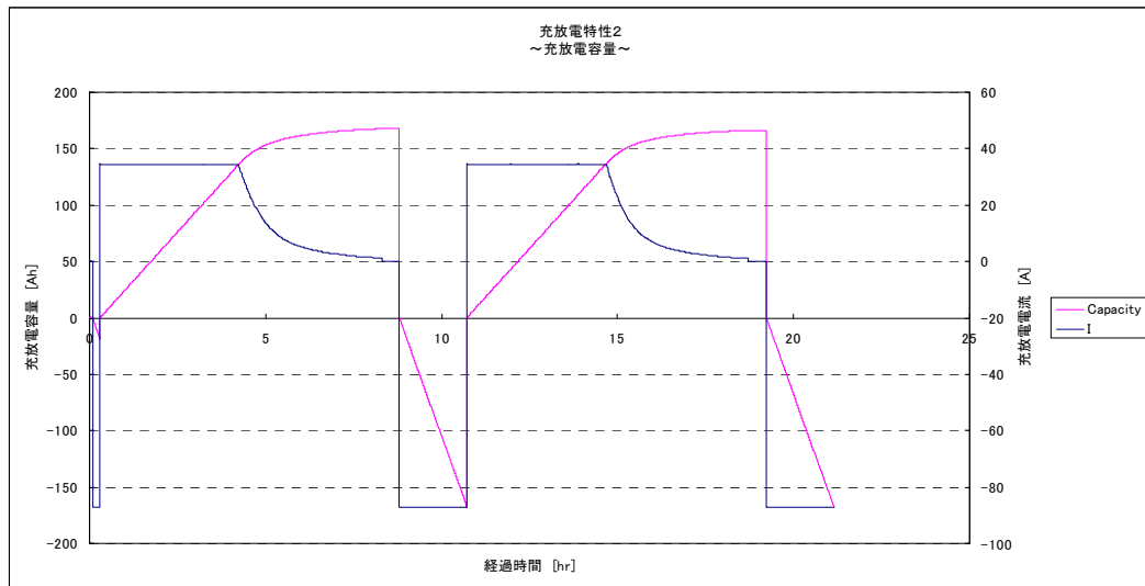
図 3.1.3.2-4 充放電特性(2/2)
