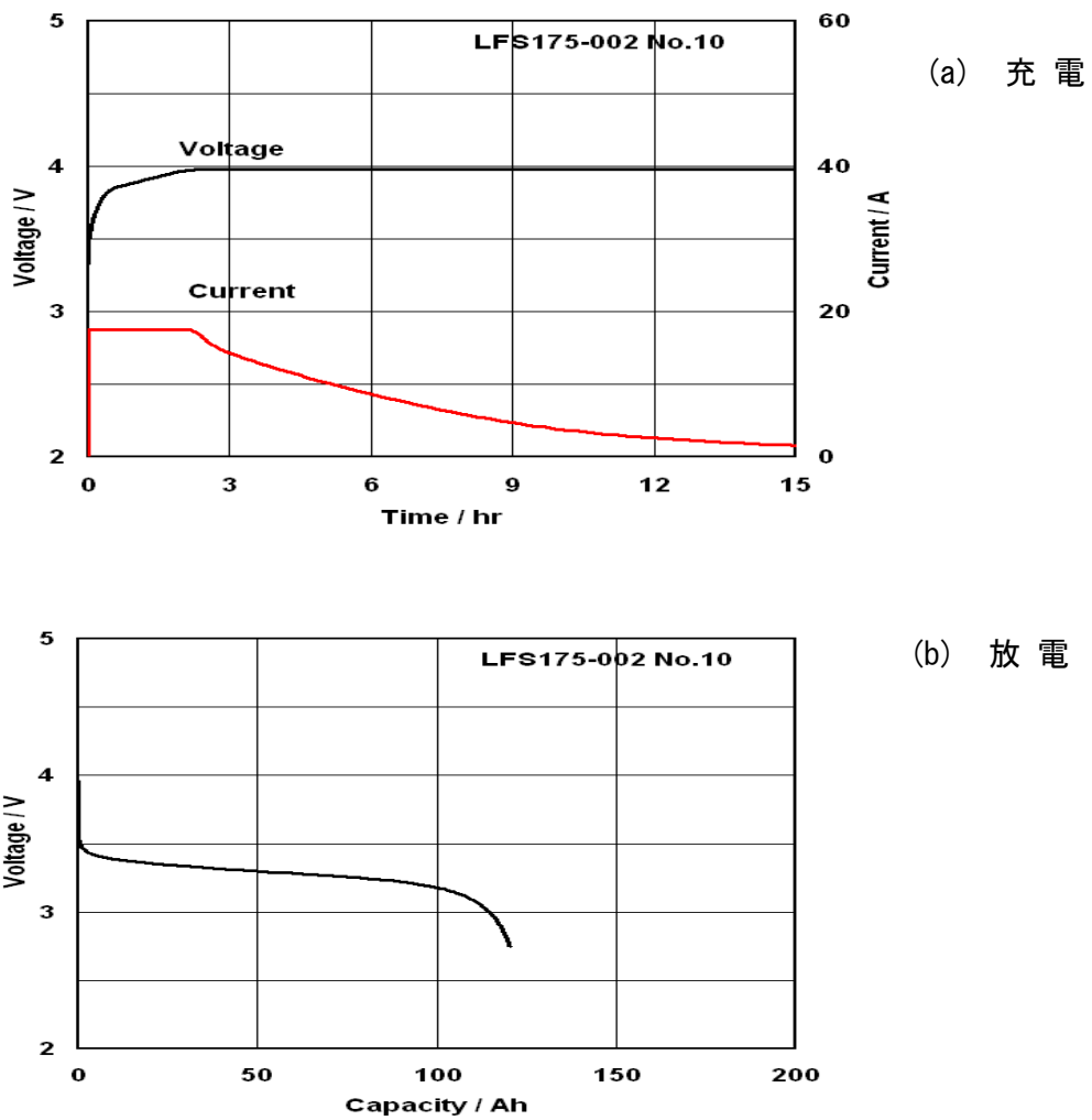
図 3.2.12.2-17 S/N010 の容量試験(15°C)での充放電曲線
