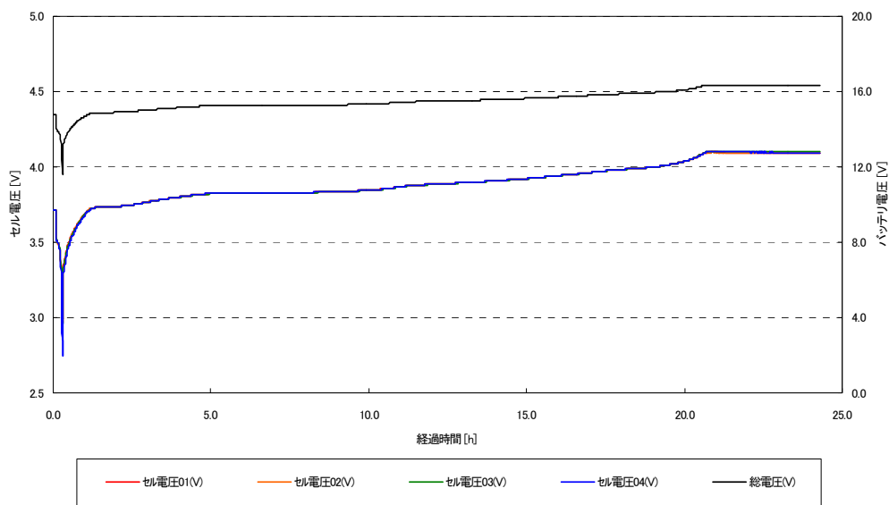
図 3. 1. 3. 5-2 過電圧保護回路動作試験時の電圧特性
