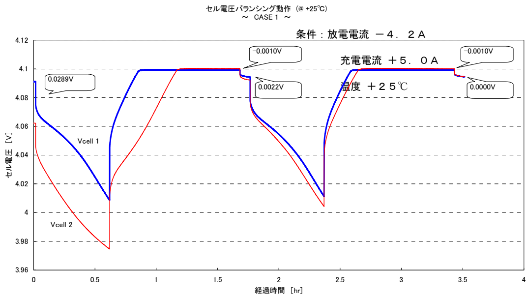
図 3.3.1-5 セル電圧バラランシング動作特性
