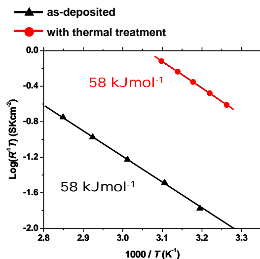
図 3.4.3-3 LiCoO 2 /LiPON 界面のイオン移動抵抗の温度依存性. 黒：熱処理なし、赤：熱処理あり.
