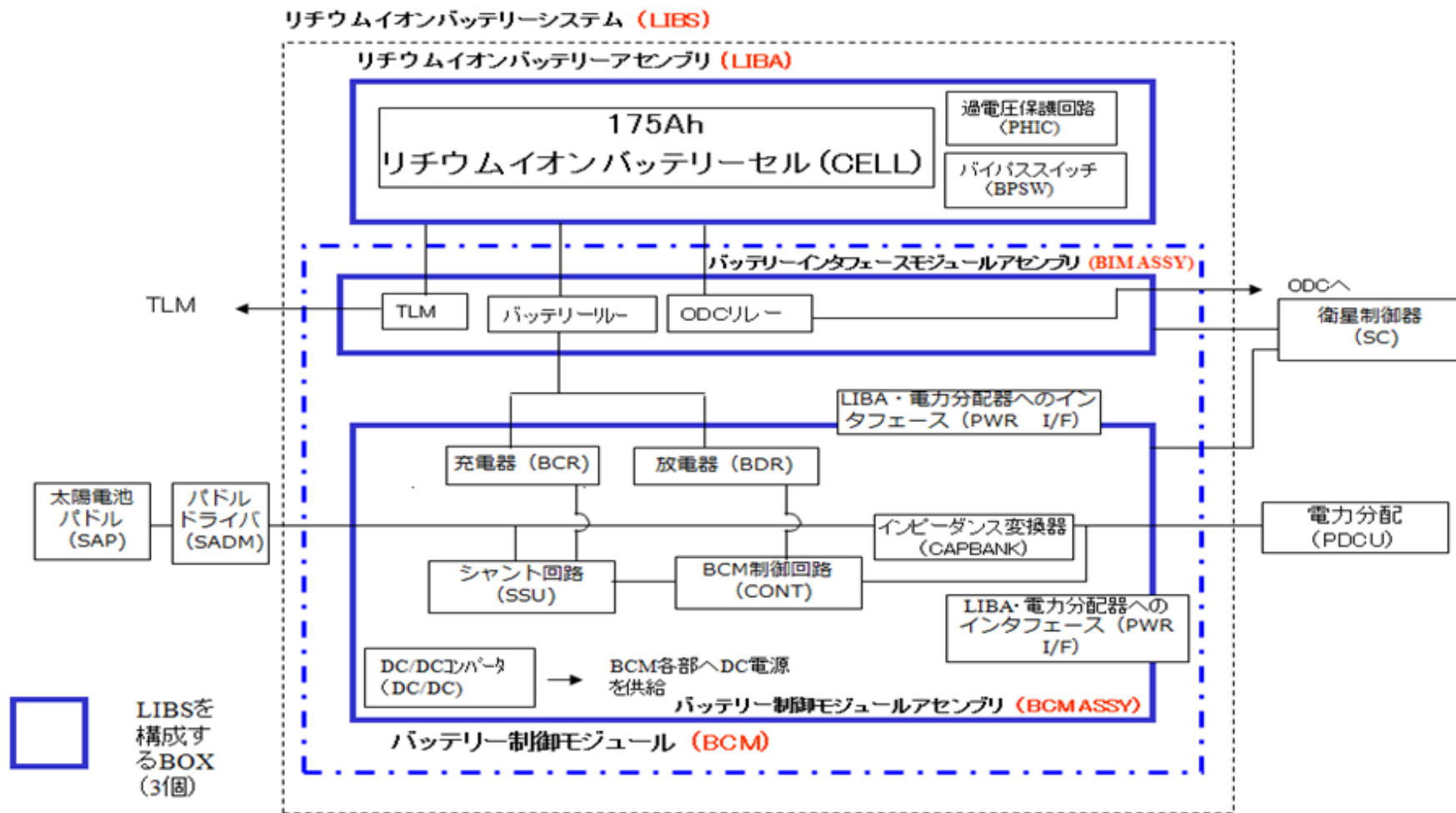
図 2.1.1-1 リチウムイオンバッテリー構成図
