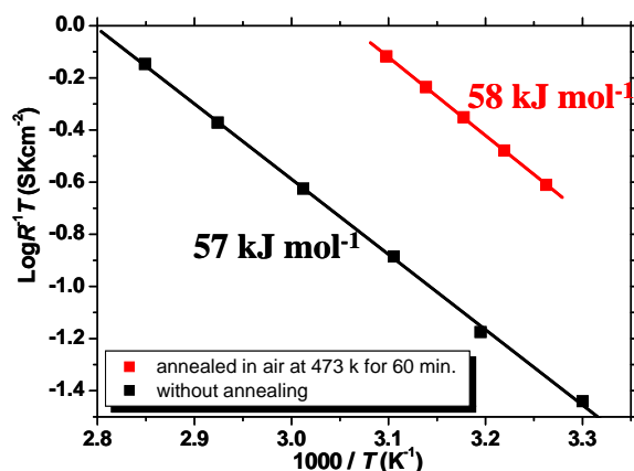
図 3. 4. 1-4 電荷移動抵抗の温度依存性 黒：熱処理前、赤：熱処理後
