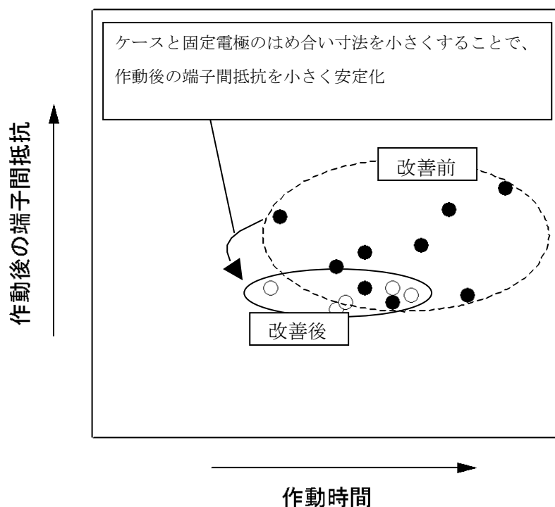
図 3.3.2-4 はめ合い寸法の大小による端子間抵抗の変化
