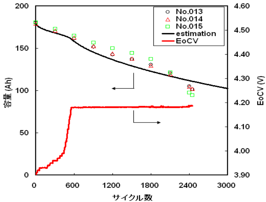
図 3.2.13.2-4 一定 EODV 試験 1 の容量確認試験での容量推移
