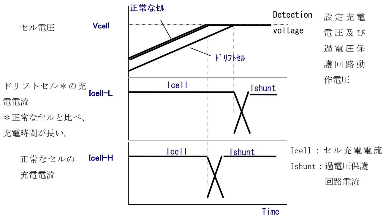
図3. 3. 1-3 バランシング機能の概略
