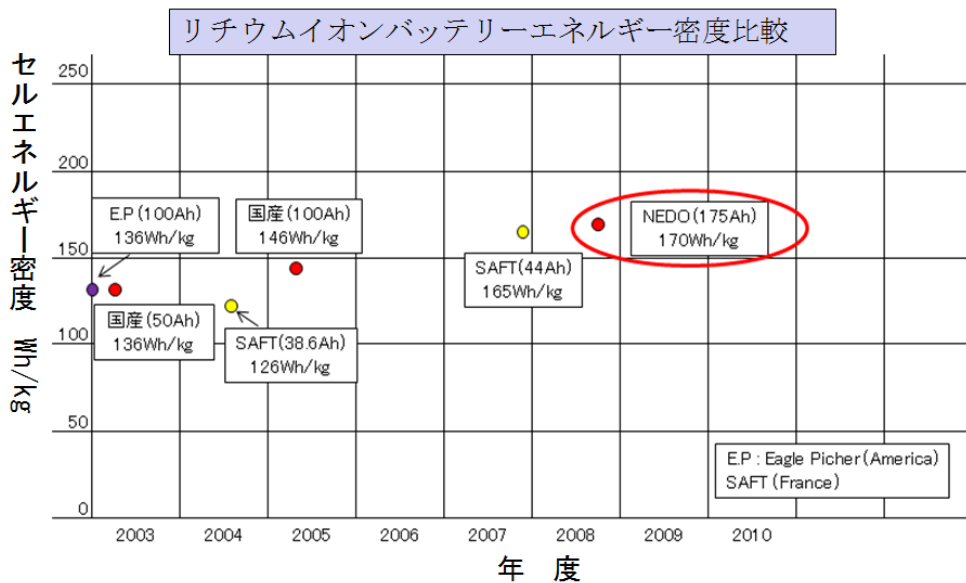
図 1.3-4 リチウムイオンバッテリーのエネルギー密度比較
