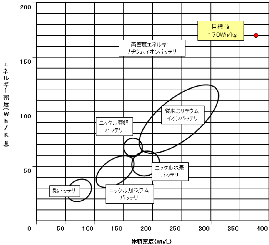
図 1.3-3 バッテリー（セル）エネルギー密度の分布
