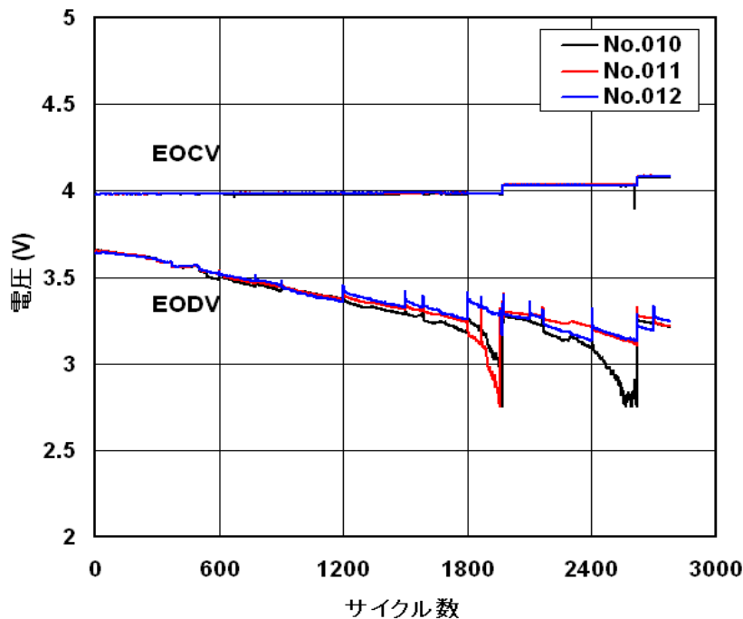
図 3.2.12.2-1 一定 EoCV 試験中の EoCV と EoDV の推移
