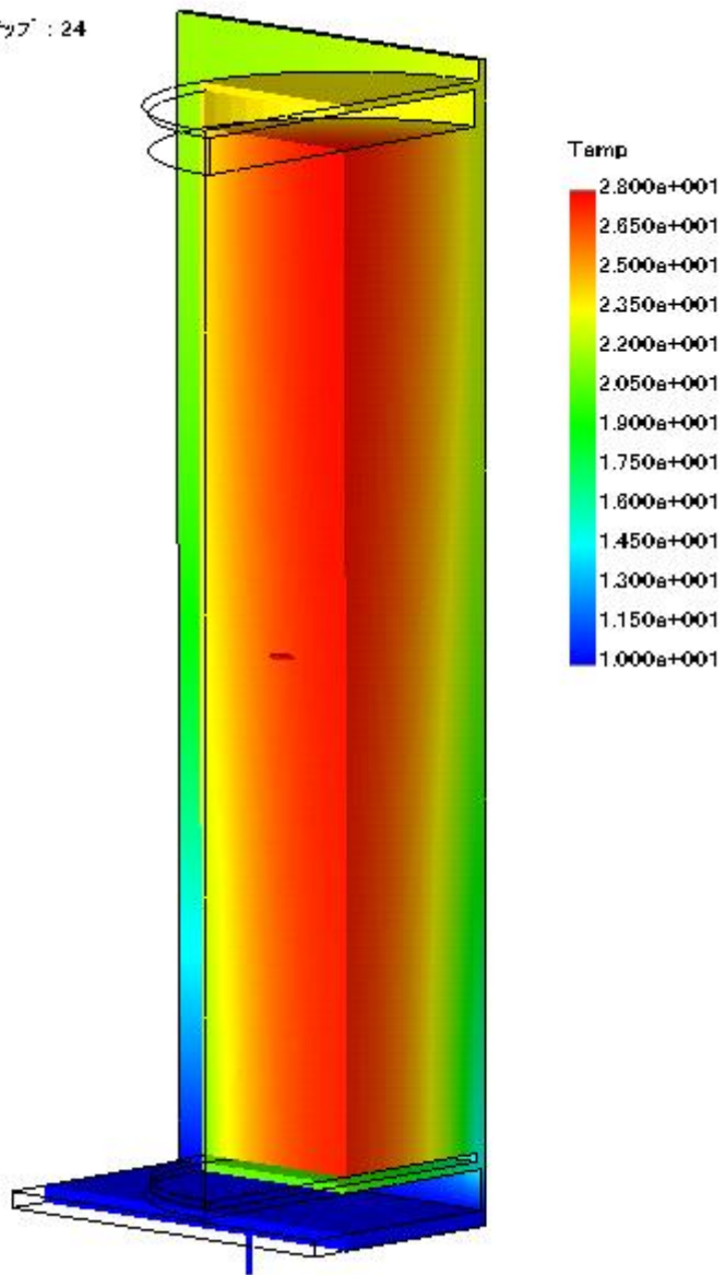
図 3. 2. 7-2 円筒形電池の熱伝導解析結果
