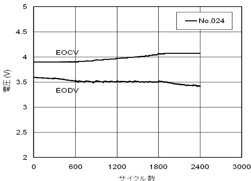
図 3.2.12.2-5 一定 EODV 試験 2 中の EOCV と EODV の推移
