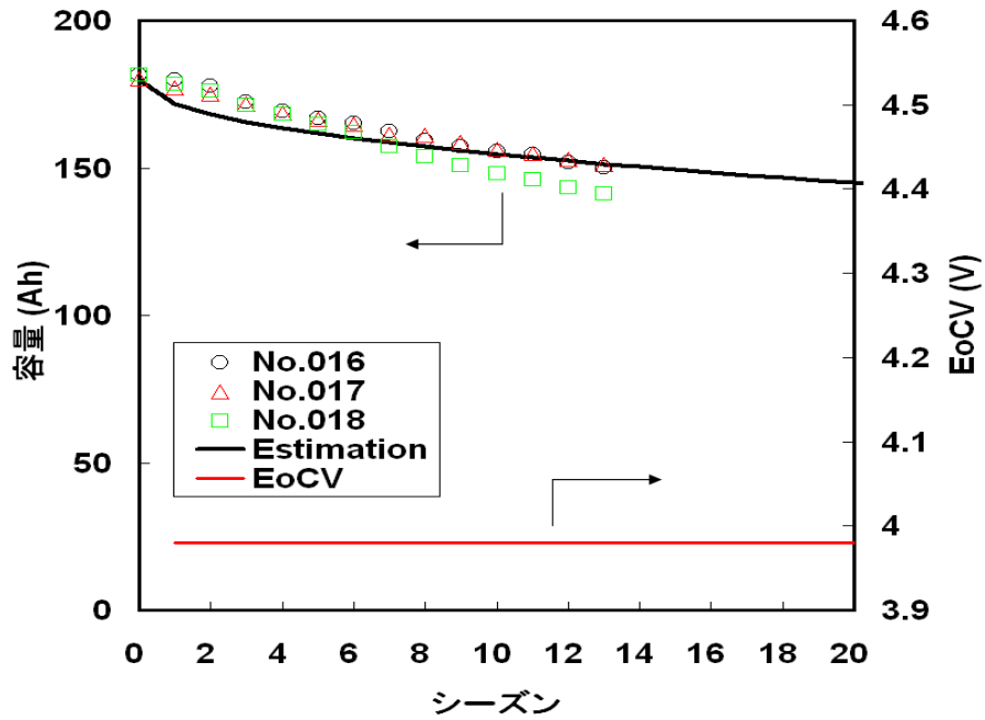
図 3. 2. 12. 2-8 一定 EOCV 静止軌道模擬試験セルの容量推移.
