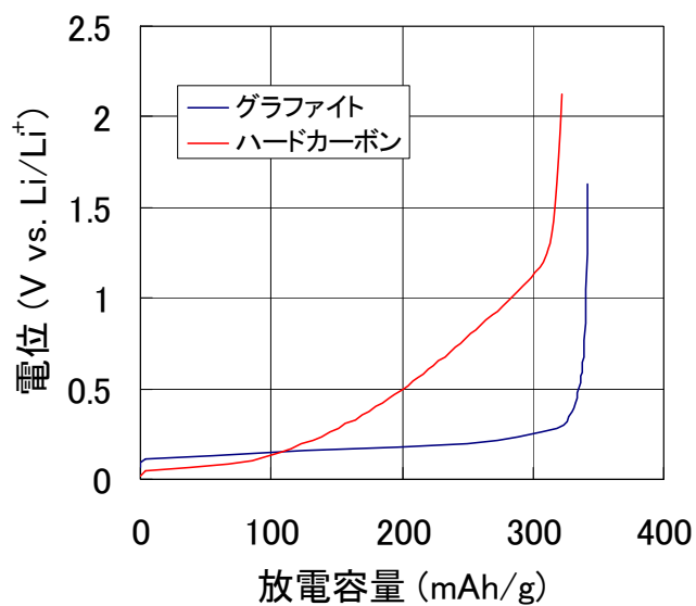
図 3.2.2-1 負極炭素材料の放電電位曲線
