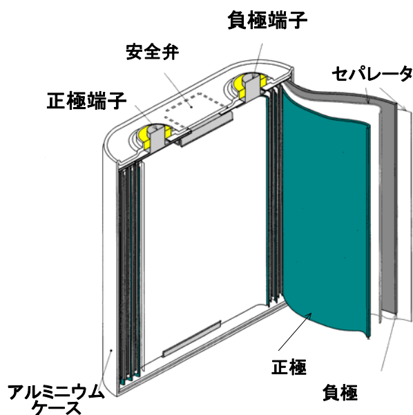
図 2. 2-1 バッテリーセルの分解図
