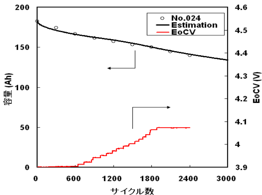
図 3.2.12.2-6 一定 EODV 試験 2 の容量確認試験での容量推移.
