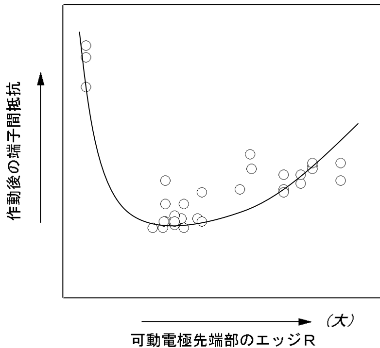
図 3.3.2-6 可動電極先端部のエッジRと作動後の端子間抵抗の関係
