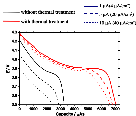
図 3.4.3-1 薄膜電池の充放電曲線.
