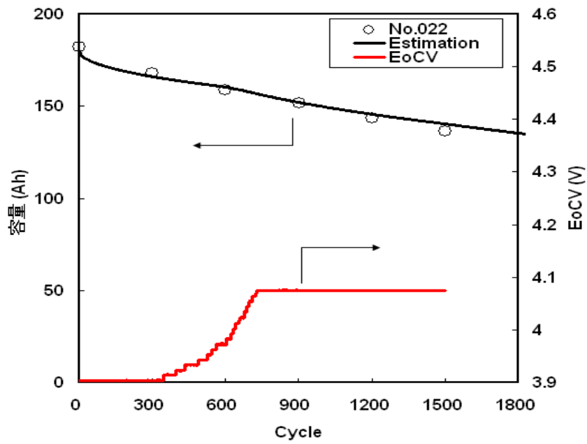
図 3. 2. 12. 2-11 準天頂衛星模擬試験①容量推移.
