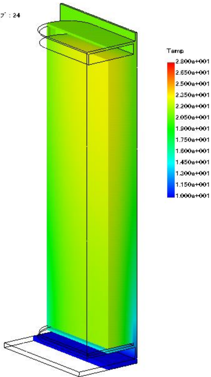
図 3. 2. 7-1 長円筒形電池の熱伝導解析結果
