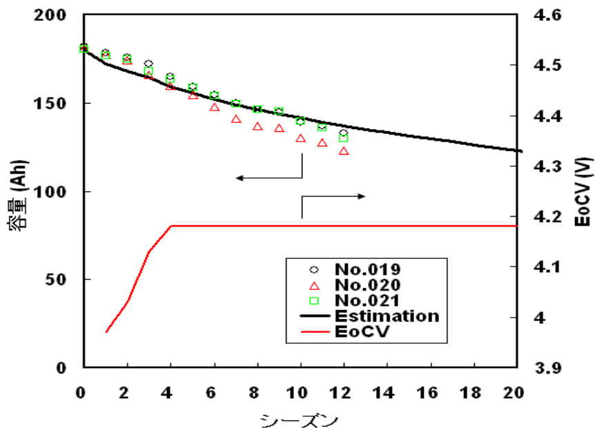
図 3.2.12.2-10 一定 EODV 静止軌道模擬試験セルの容量推移.
