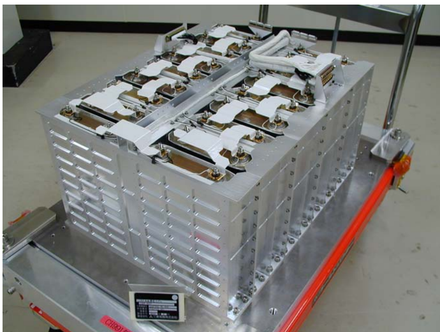
図 2.1-1 バッテリーアセンブリ（開発モデル：18 セル）
