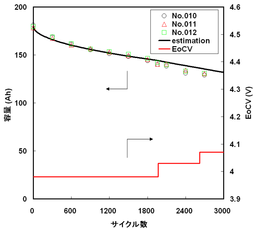
図 3. 2. 12. 2-2 一定 EOCV 試験の容量確認試験での容量
