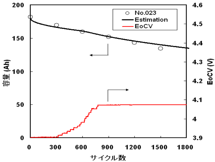
図 3. 2. 12. 2-12 準天頂衛星模擬試験②容量推移.
