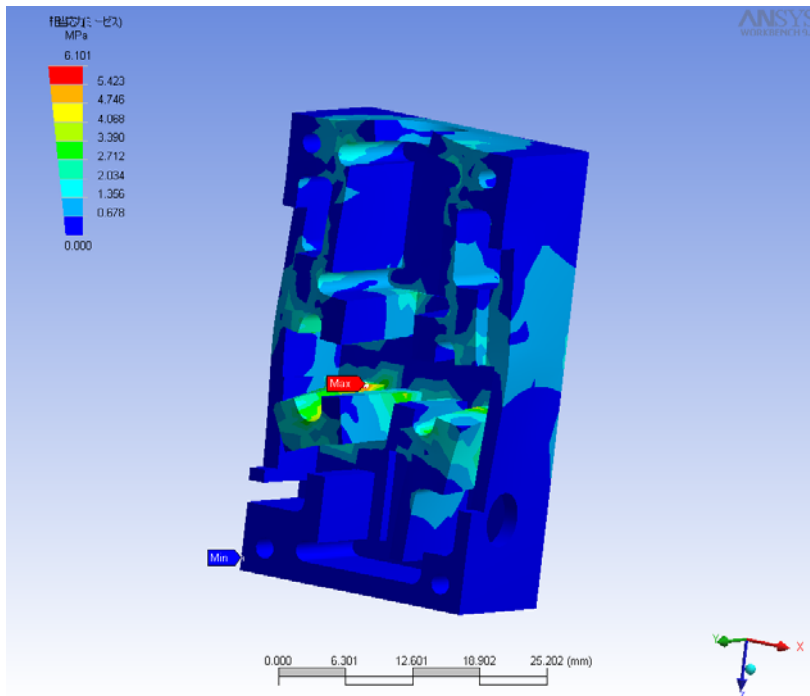
図 3.3.2-9 相当応力 (バイパススイッチ作動後)
