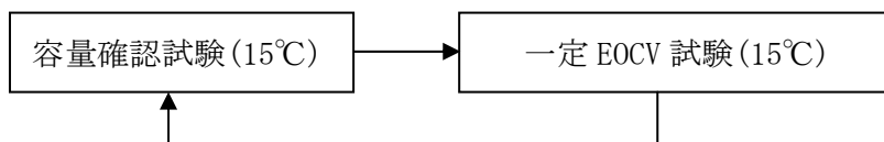
図 3.2.12.1-2 一定 EOCV 試験フロー
