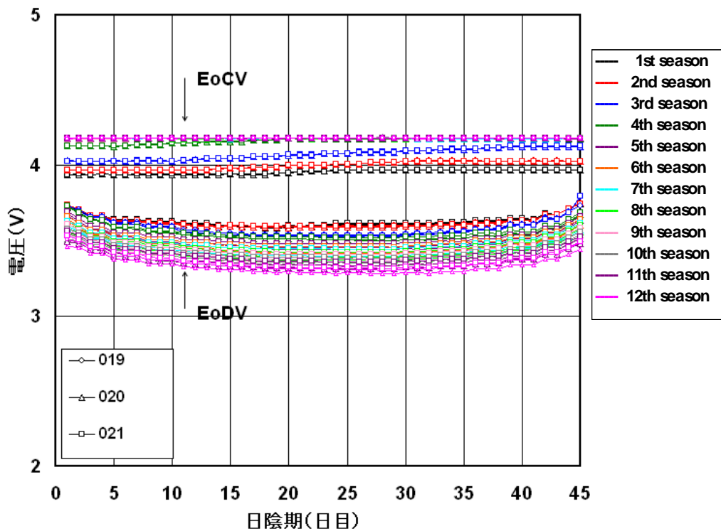
図 3.2.12.2-9 一定 EODV 静止軌道模擬試験セルの EOCV、EODV の推移。
