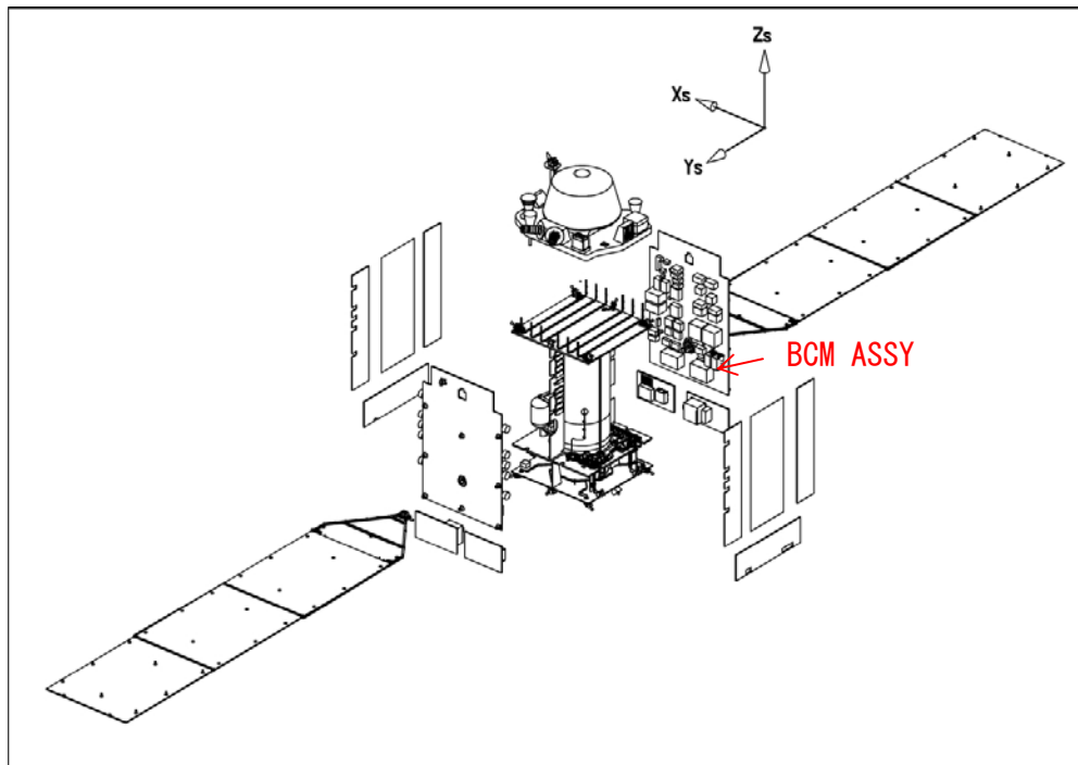
図 3.1.6.2-2 外部搭載機器および構体パネル内構成図 (図 JAXA 提供)
