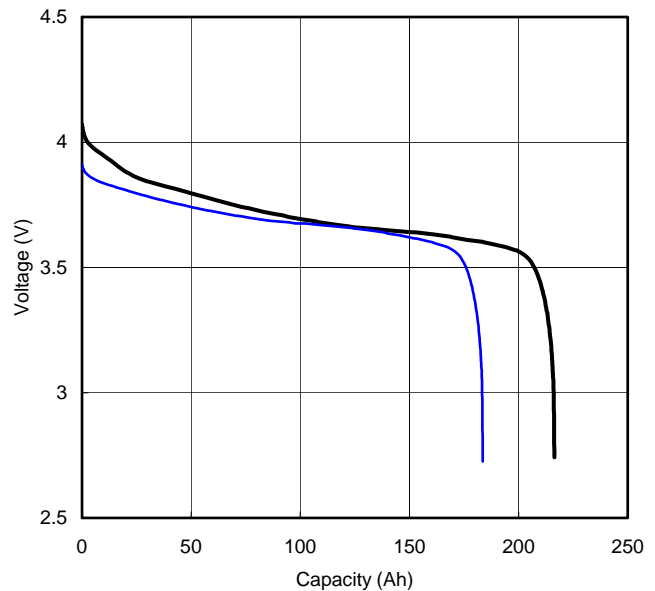
図 3.2.9-5 セルの容量確認データ
