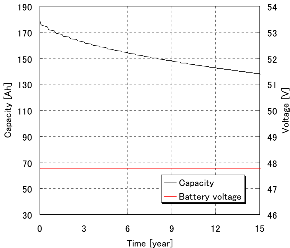
図3.1.3.6-5 静止衛星模擬シミュレーション
