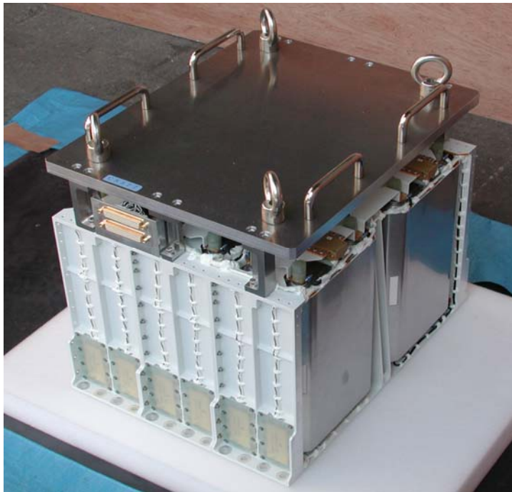
図 3.1.3.4-1 LIBA 安全性評価モデル
