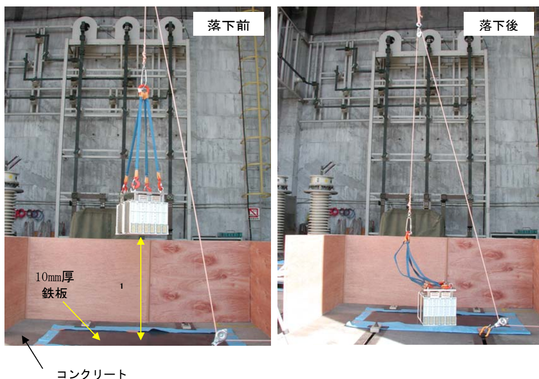
図 3.1.3.4-3 落下試験状況の外観
