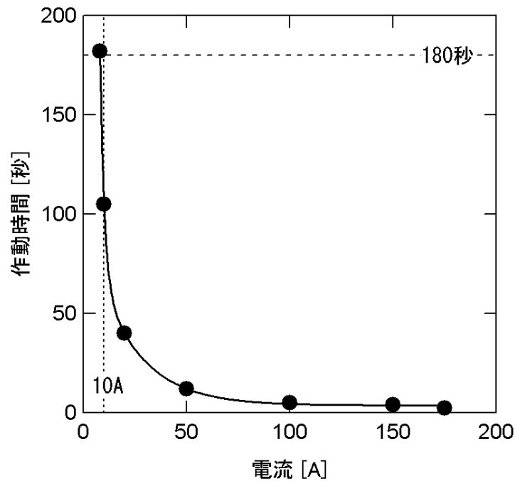
図 3.3.2-2 電流と作動時間の関係
