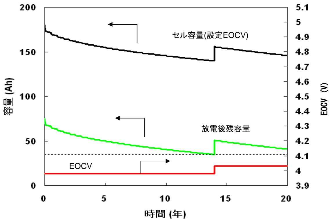
図 3.2.12.2-15 準天頂衛星模擬試験条件における寿命シミュレーション
