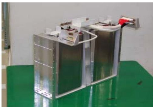
図 3.1.1-1 試作4セルモジュール（シェル構造）
