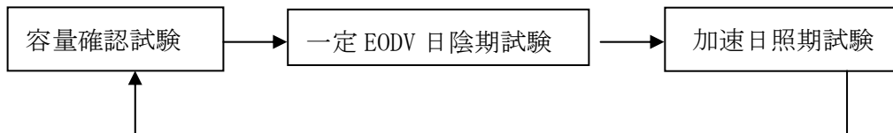
図 3.2.12.1-5 一定 EODV 静止軌道衛星模擬試験フロー
