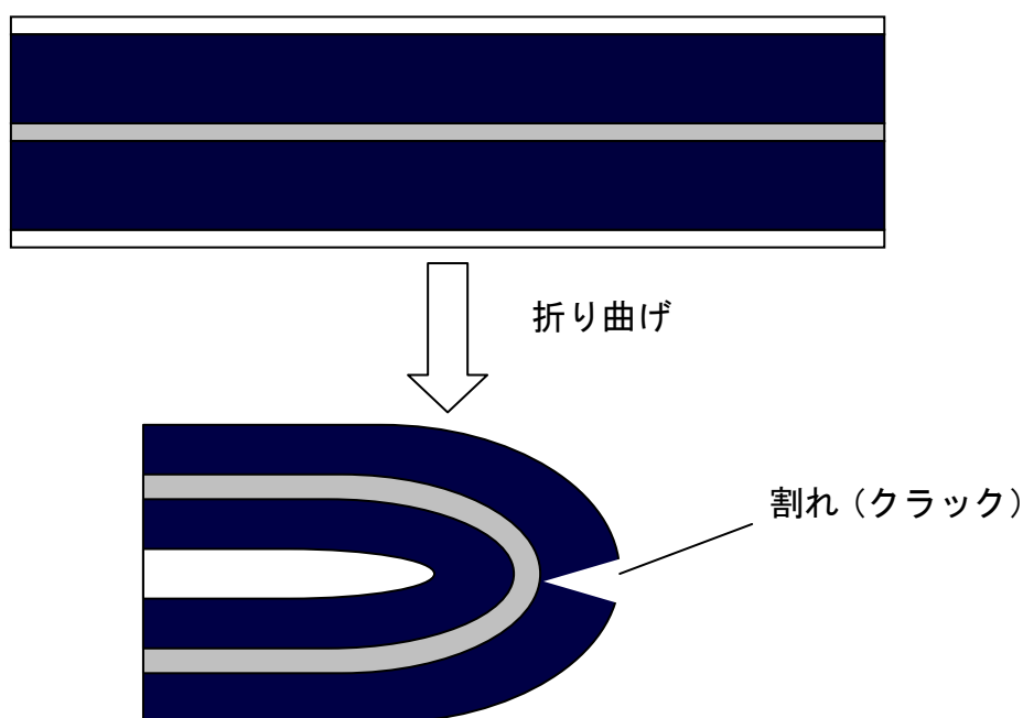
図 3.2.4-2 折り曲げ時の応力による活物質の割れ
