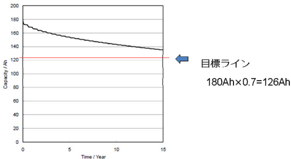
図 3.2.12.2-16 静止衛星模擬試験条件に於ける寿命シミュレーション
