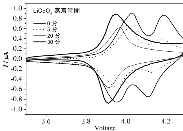
図 3.4.5-1 HT-Co LiMn 2 O 4 (5, 20, 30) / LiPON / Li薄膜電池の電位挿引曲線。
