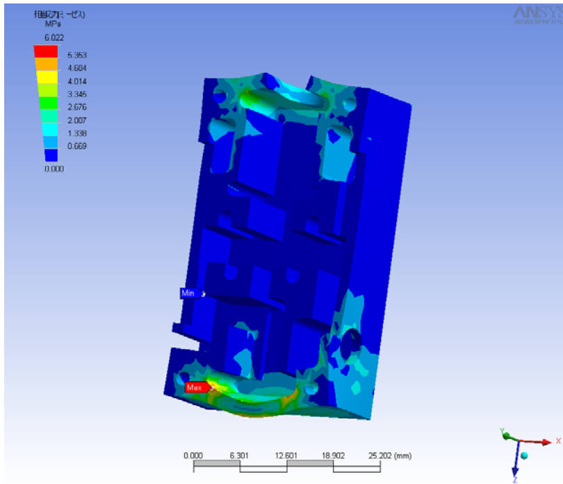
図 3.3.2-8 相当応力 (バイパススイッチ作動前)
