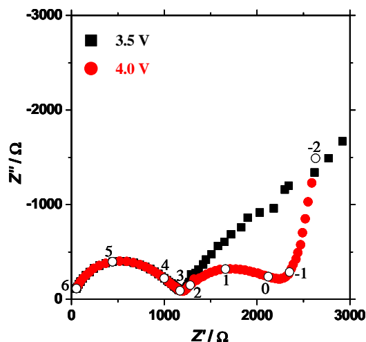
図 3.4.3-2 薄膜電池の Cole-Cole plot. 黒：3.5V、赤：4.0V. 白抜きデータポイントは 10 4 Hz で測定された点.
