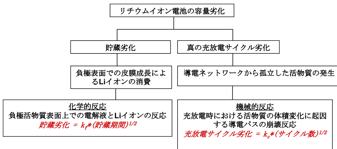
図 3.2.9-6 リチウムイオン電池容量低下の体系
