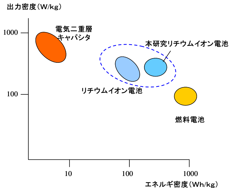
図 4.1.5.2.4-1 エネルギー密度/出力密度関係図
