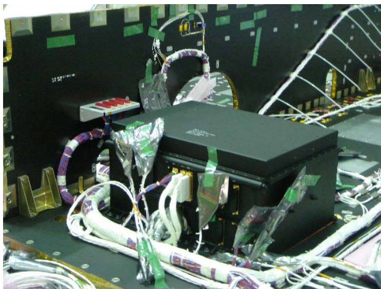
図 3.1.6.2-3 BCM ASSY の衛星システムパネルの搭載写真 (図 JAXA 提供)
