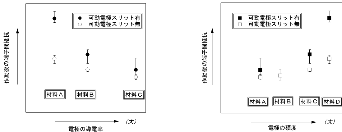
図 3. 3. 2-5 電極の形状と端子間抵抗の関係
