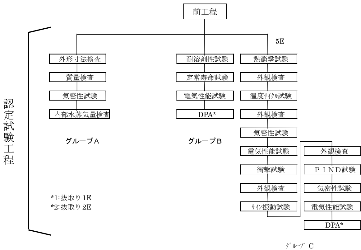
図 3.3.1.2-1 認定試験フロー
