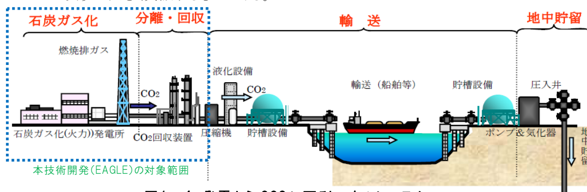
図1-4 発電からCCSに至るトータルシステム
