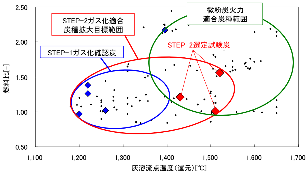
図3-7 EAGLE 試験炭性状分布図
