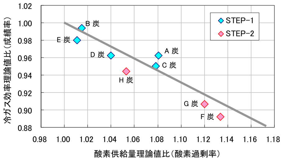
図3-8 ガス化性能図(酸素供給量および冷ガス効率の理論値比)
