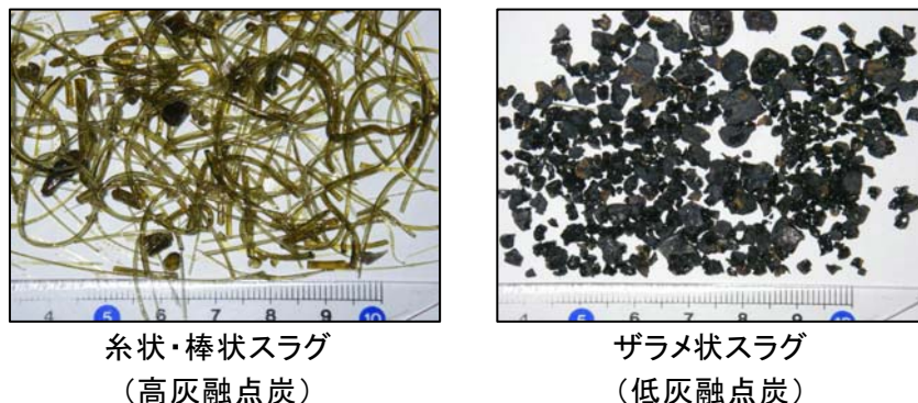
図3-9 EAGLE スラグの外観
