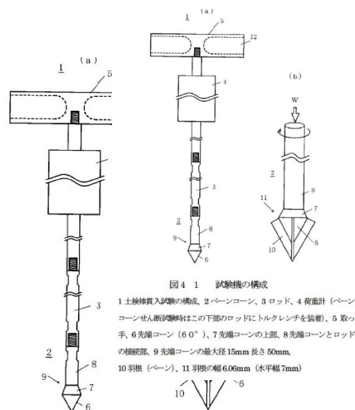
図4 1 試験機の構成
