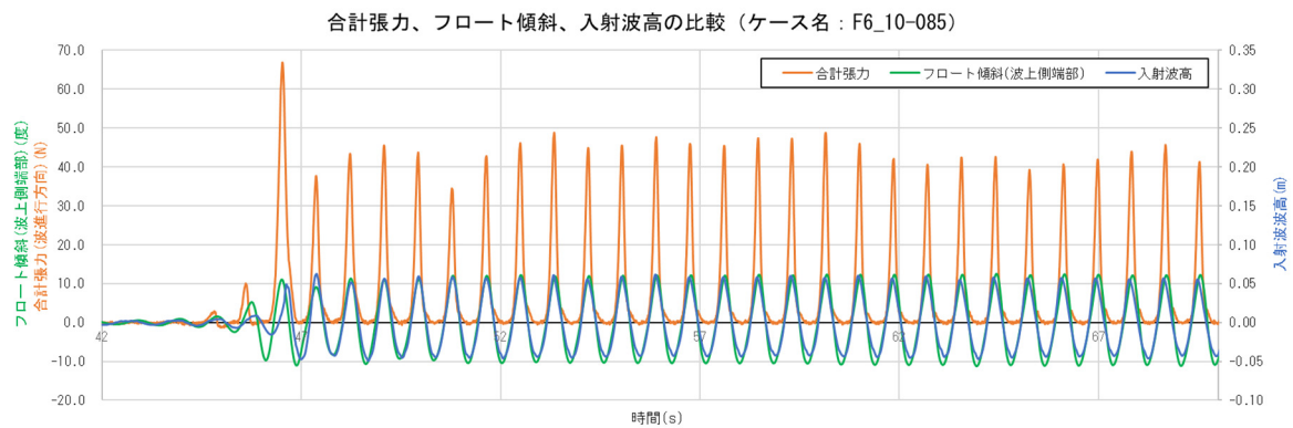
図 5-7 被災波相当波浪（F6_10-085）における合計張力、フロート傾斜、入射波高の比較結果
