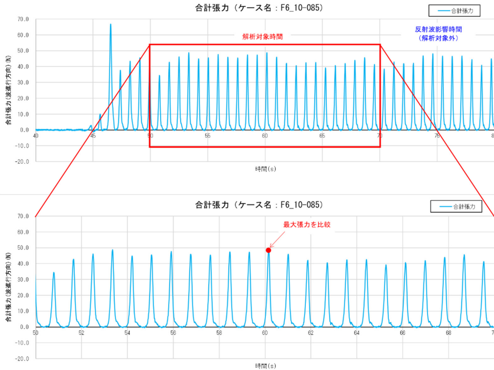
図 5-1 張力の解析対象時間（ケース名：F6_10-085）
