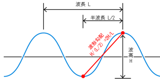
図 5-17 波形勾配
