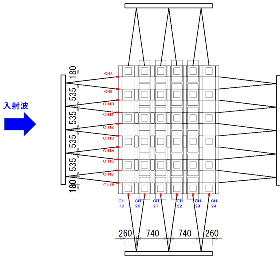
図 4-3 張力計（リングゲージ）設置箇所
