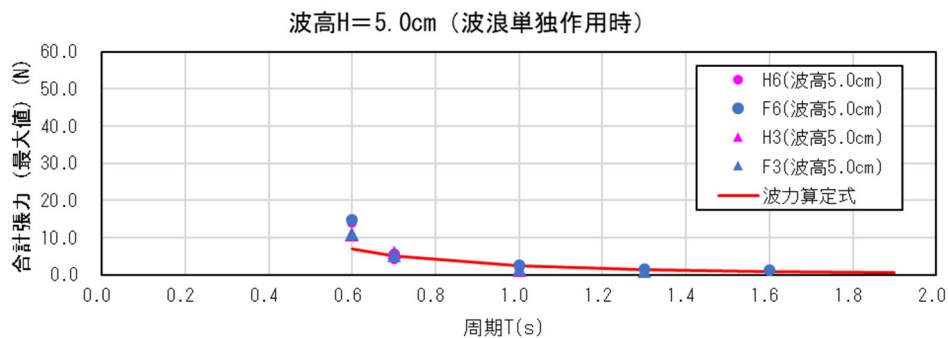
図 5-5 計測値と計算値の比較結果 (波高 H=5.0cm)
