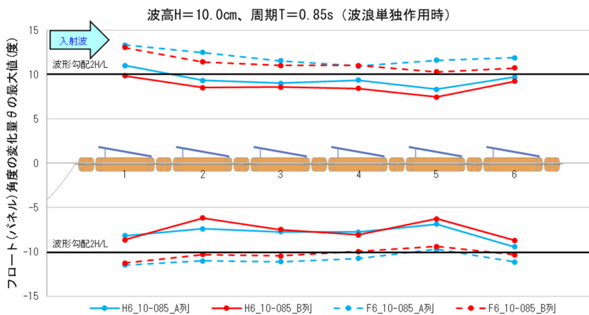
図 5-20 短周期のケースにおけるフロート(パネル)の傾斜角と波形勾配の比較(波高 10.0cm)
