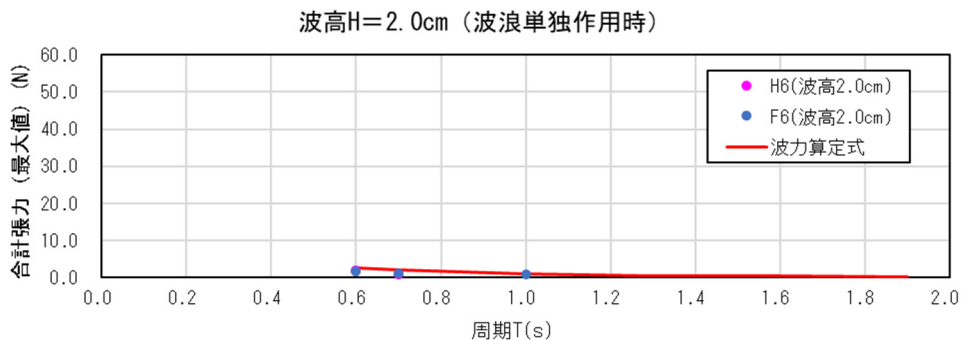
図 5-4 計測値と計算値の比較結果 (波高 H=2.0cm)
