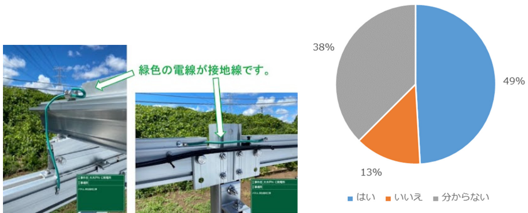
図 3-24 太陽電池モジュールと架台は接地線で接続されているか（n=112 件）
