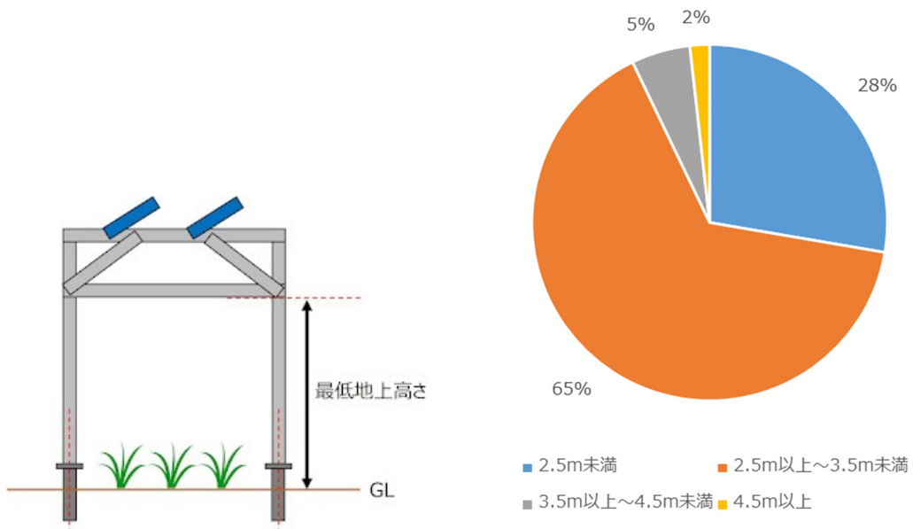
図 3-6 地面（GL 部）から最低地上高さ（n=112 件）
