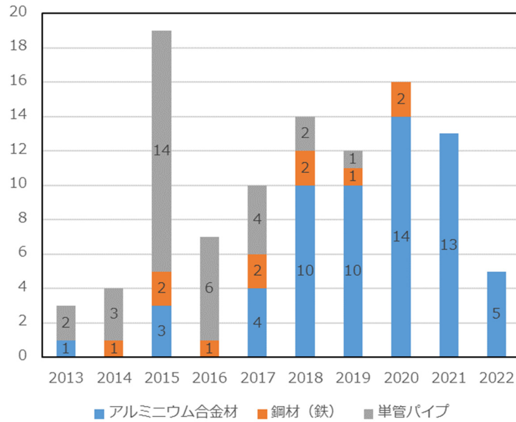
図 3-9 架台の種類と設置時期
