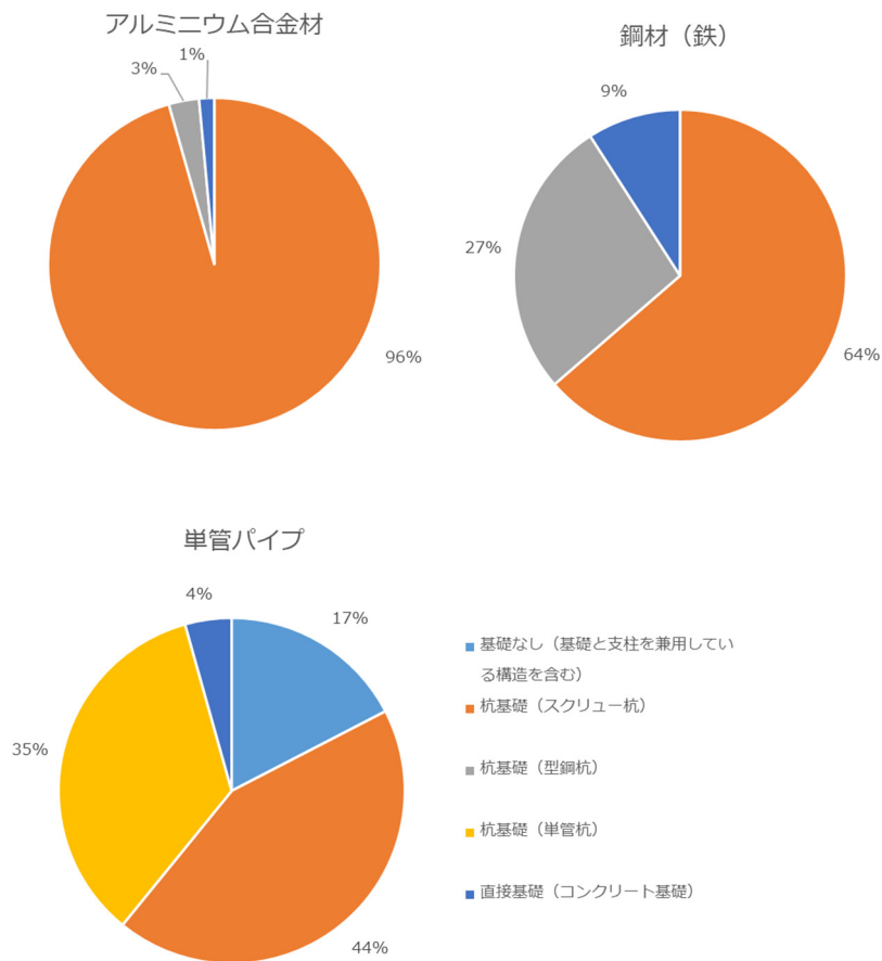
図 3-10・基礎構造と架台材料との関係
