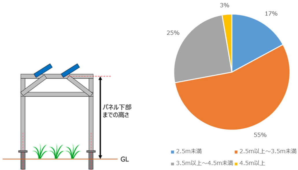
図 3-5 地面（GL 部）から太陽電池アレイ下部までの平均高さ（n=112 件）
