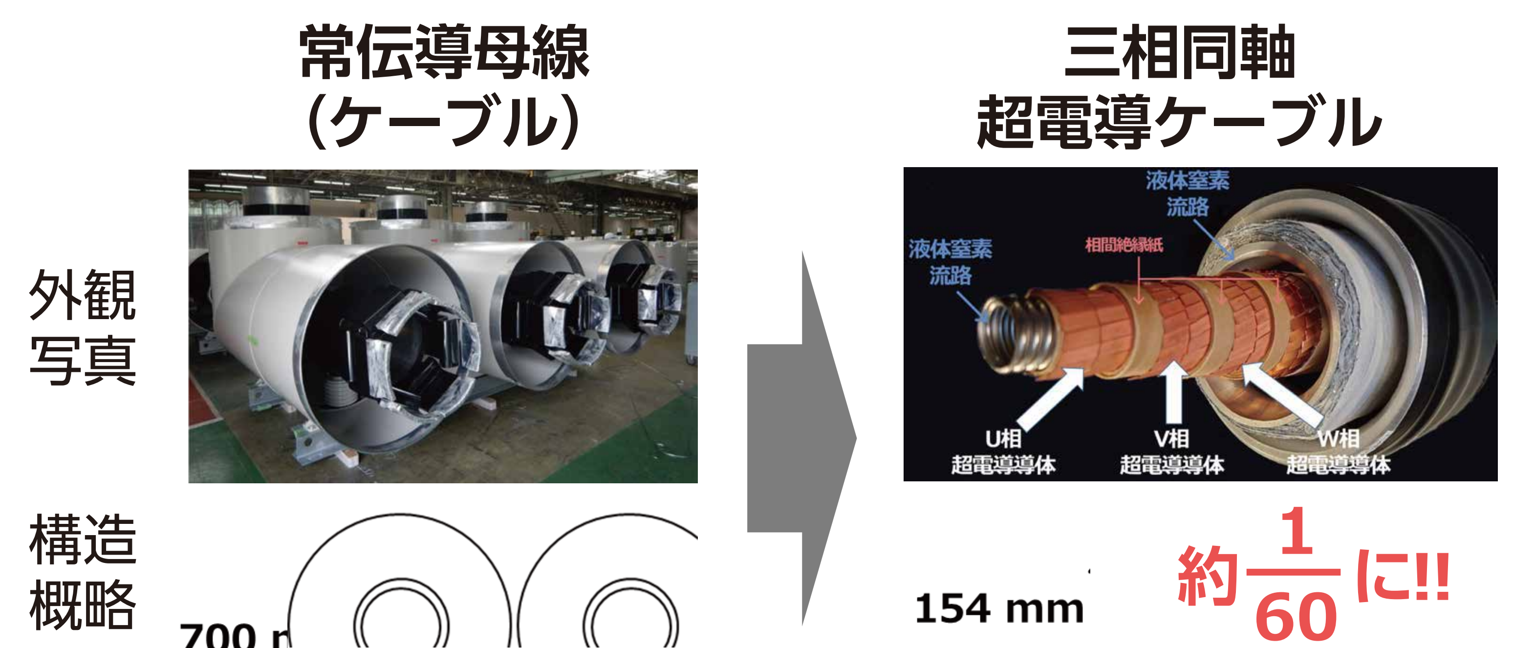
常伝導ケーブルと三相同軸超電導ケーブルの比較
