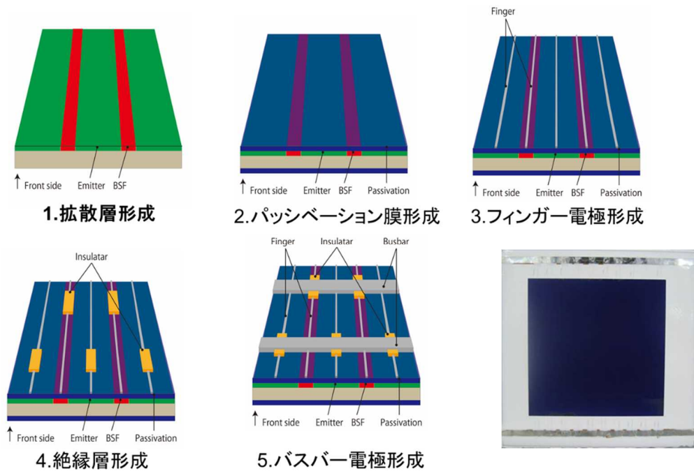
図Ⅲ-2-(ニ)-B-13 両面受光-裏面電極型セルの作製プロセスと裏面側の写真(右下)
