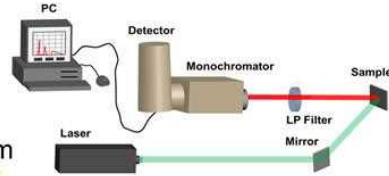
図 III-2-(二)-A-8 室温発光活性化 PL (RT-PL) 法の概要。
