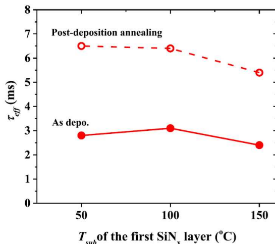
図Ⅲ-2-(ニ)-C-6 第一層堆積時の基板温度と \tau_{\text{eff}} の関係
