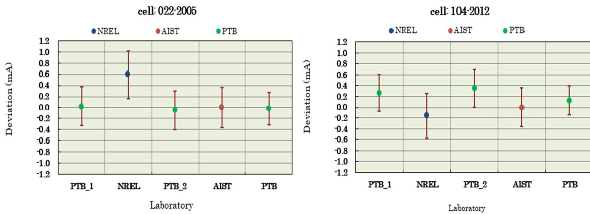
図Ⅲ-2-(ホ)-A-I-1-13 WPVS根幹ラボ間での比較校正 (上図 器物022-2005, 下図 器物104-2012)
