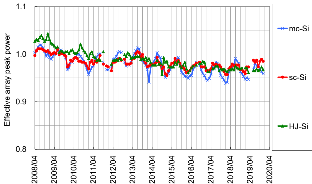
図III-2-(ホ)-C-5 アレイ実効最大出力係数の算出結果
