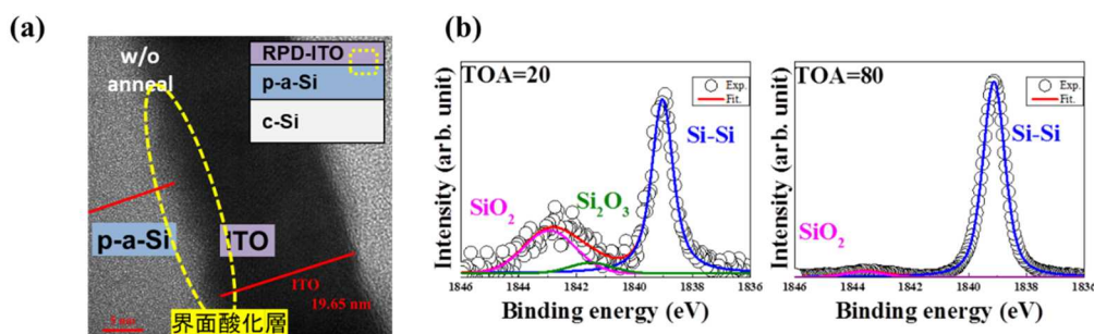
図 III-2-(二)-A-21 (a) RPD-ITO/p-a-Si 界面の断面 TEM 像、および、(b) Si 1s コアレベルスペクトルの光電子取出し角 (TOA) 依存性。
