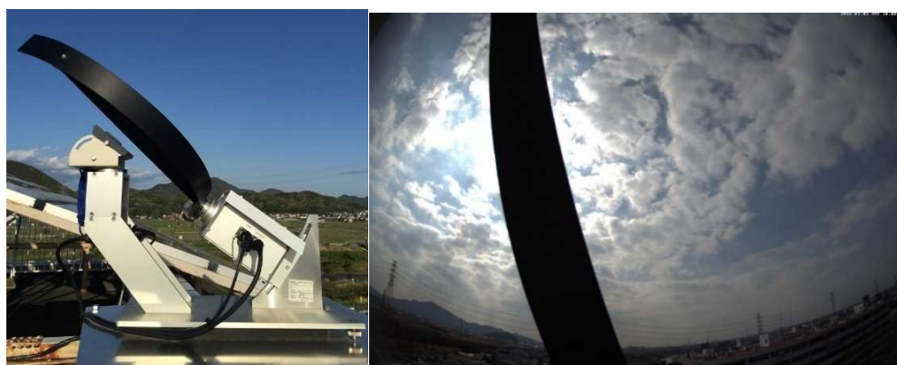
図Ⅲ-2-(ホ)-A-Ⅲ-2 シャドーブレード付き上空カメラの外観(左図)とこのカメラによって捉えられた雲および日射の様子(2016年3月6日10時)
