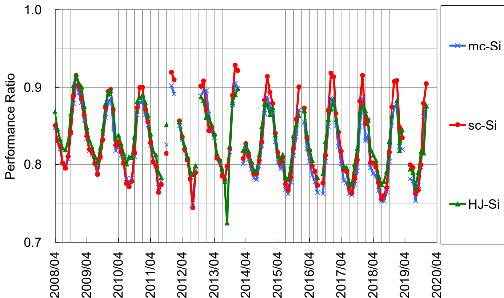
図III-2-(ホ)-C-4 システム出力係数の算出結果
