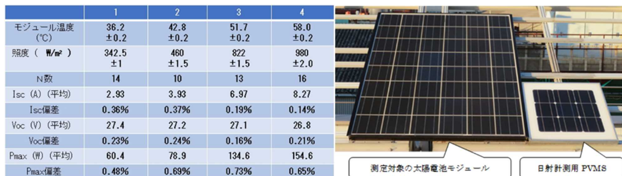
図Ⅲ-2-(ホ)-A-VI-1 (左) JET 電力技術試験所屋上に設置した結晶シリコン系モジュールと PVMS (右) 短絡電流・開放電圧・最大電力の測定再現性精度 (JET 屋上結晶シリコン系モジュール)
