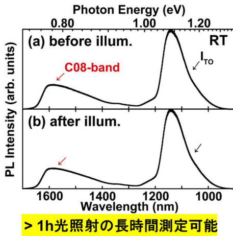
図 III-2-(二)-A-9 MCZ Si 結晶の室温 PL スペクトル (炭素濃度: 1 \times 10^{15} \text{ cm}^{-3} ) : (a) 2 MeV 電子線照射直後、および、(b) 引き続き 1 hr レーザー照射後。
