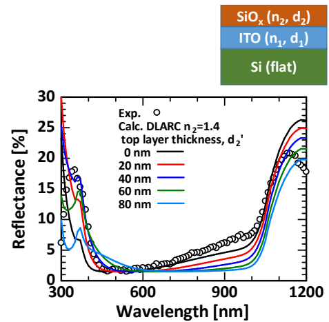
図 III-2-(二)-A-46 ITO 単層膜の反射率の実測結果および 2 層化した場合の反射率のシミュレーション結果
