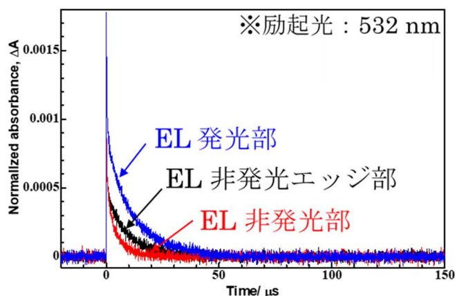
図Ⅲ-2-(ホ)-E-7 TAS法により測定したキャリア減衰曲線
