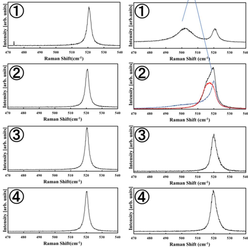
図Ⅲ-2-(ニ)-A-16 加工方向に沿った Raman スペクトルの比較。番号は、図Ⅲ-2-(ニ)-A-15 において番号で示された反射率分布測定位置に対応する。
