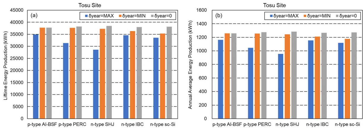
図Ⅲ-2-(ホ)-B-23 各種結晶 Si 太陽電池の (左) 30 年間の生涯発電量、(右) 1 年当たりの年平均発電量
