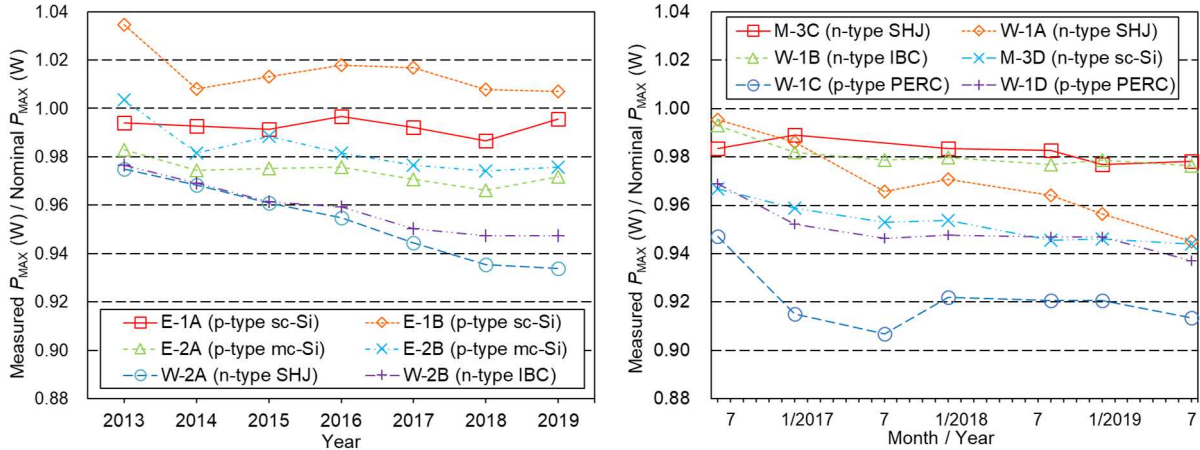
図Ⅲ-2-(ホ)-B-21 (左) 2012 年 12 月、(右) 2016 年 6 月に導入した結晶 Si 太陽電池の室内測定出力の推移
