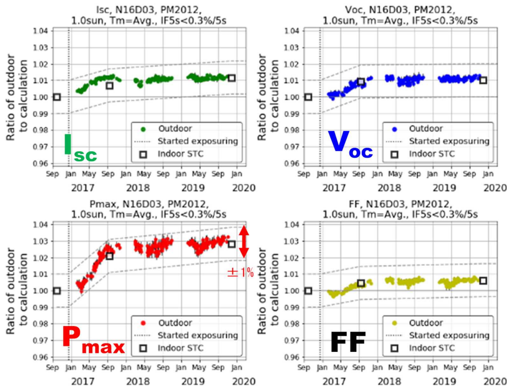
図III-2-(ホ)-A-I-2-4 長期（約3年間）の市販結晶シリコン太陽電池モジュール屋外性能測定結果。縦軸は I_{sc} , V_{oc} , P_{max} , FF 屋外計測値の測定開始前屋内測定値との比率。□印は屋内測定結果。
