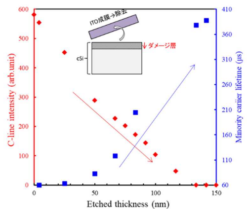
図 III-2-(ニ)-A-24 C-line 強度、および、ライフタイムのエッチング深さ依存性
