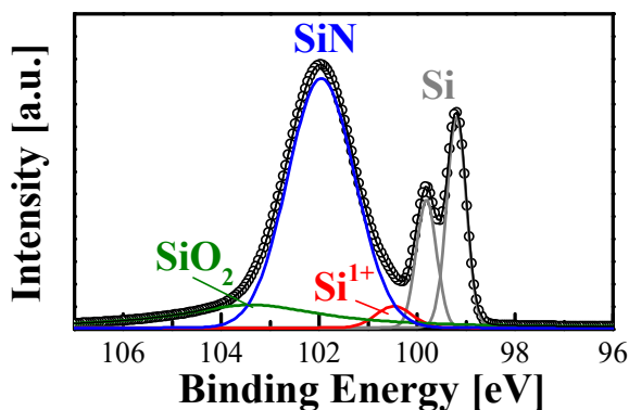
図III-2-(二)-A-19 SPring-8、硬 X 線光電子分光 (HAXPES) 法によって測定した、SiN x 膜界面における化学結合状態による Si2p ピークの分裂
