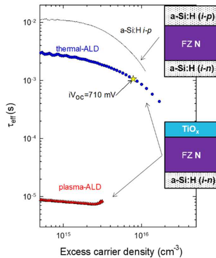
図Ⅲ-2-(ニ)-E-2. 結晶 Si 基板の片面をプラズマ ALD TiO x (赤) またはサーマル ALD TiO x (青) でパッシベーションしたサンプルの少数キャリアライフタイムの注入キャリア濃度依存性。
