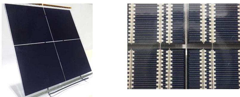
図Ⅲ-2-(ニ)-B-15 両面受光-裏面電極型セルを用いて作製したモジュール(セル：4枚) 表面側の写真(右)および裏面側の写真(左)。細線ワイヤを用いてセル間の配線を行っている。
