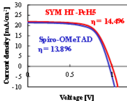
(b) 太陽電池特性
