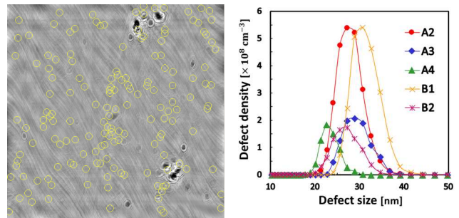
図Ⅲ-2-(二)-A-4 1100° C、3時間の熱処理後の(a) SIRMによる赤外後方散乱像と散乱体の検出結果(黄色の円)および(b) 欠陥のサイズ分布
