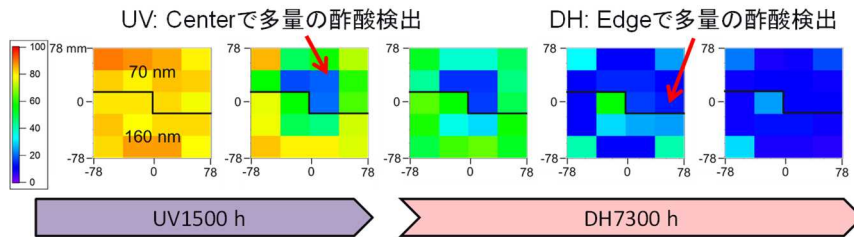
図 III-2-(ホ)-B-14 30%RH UV+DH 試験中における反射率のマッピング
