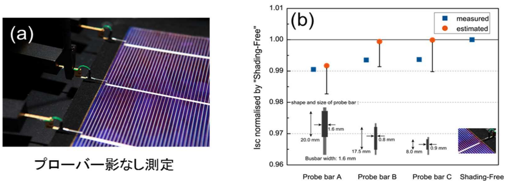
III-2-(ホ)-A-I-1-1 (a) プローブを使用したベアセル影なし測定の測定配置図（写真）、(b) 各種プローブバー影による I_{sc} への影響の実験(measured)と計算結果(estimated)の比較。影なし測定時の I_{sc} を 1.0（リファレンス）として図示
