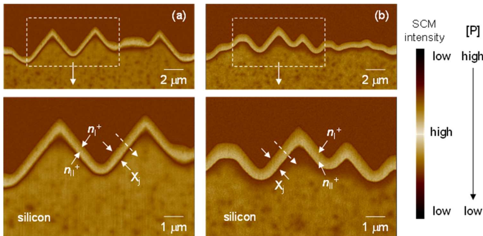
図Ⅲ-2-(二)-B-17 Al-BSF 型セルのリン注入の活性化アニールを(a)窒素雰囲気と(b)ウェット酸化雰囲気で行ったときの走査型容量顕微鏡像。 X_j が接合深さである。
