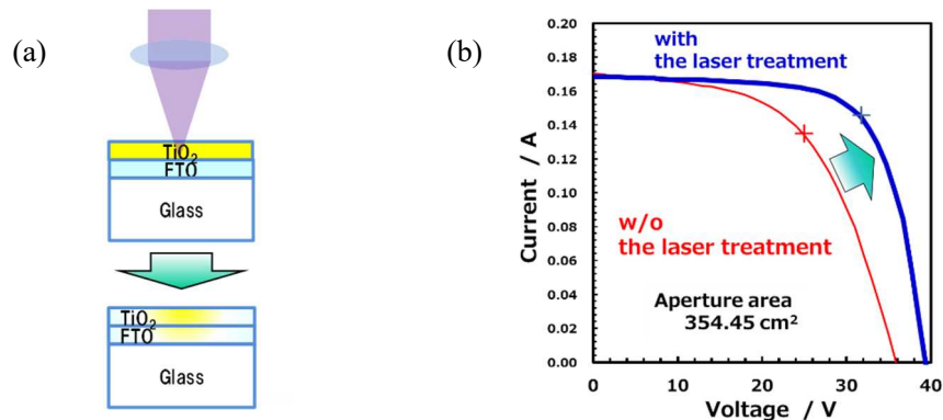
図Ⅲ-2-(ハ)-A-15 紫外線レーザー照射によるコンタクト抵抗低減の模式図(a)と紫外線レーザー照射有無の20cm角モジュールの電流-電圧特性(b)
