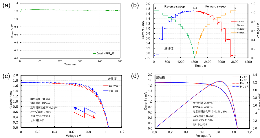
図III-2-(ハ)-F-8 MPPT 法のアルゴリズム改良による信頼度向上 (a) MPPT 法による長時間計測, (b) 元データへ変換, (c) J - V 曲線への変換, (d) (c) の収束値で近似 (ヒステリシスの解消)
