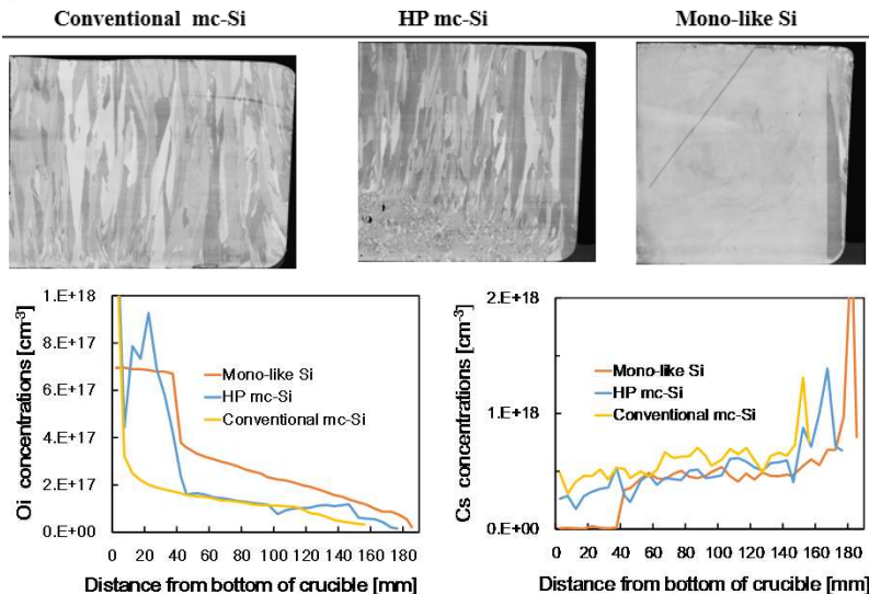
図 III-2-(二)-A-11 従来型多結晶、HP 多結晶、擬似単結晶シリコンの試料断面。インゴットから結晶成長方向に平行にスライスした。
