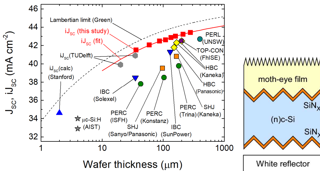
図 III-2-(二)-B-1. 実験および解析的に求めた iJ_{sc} のウエハ厚依存性。比較のため、各種文献に記載された J_{sc} および iJ_{sc} も記載した。右図は今回 iJ_{sc} 評価用に用いた模擬太陽電池サンプルの模式図。
