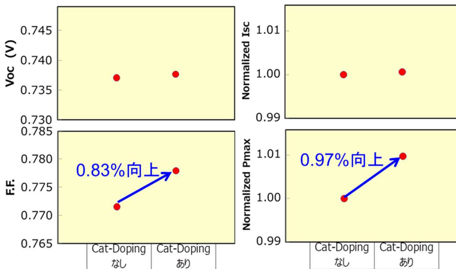
図Ⅲ-2-(ニ)-C-13 P Cat ドーピングを行った SHJ セルと比較用セルの発電性能
