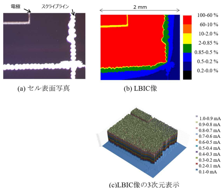
図 III-2-(ホ)-A-I-1-7 CIGS 太陽電池スクライブ線近傍の (a)セル表面写真 (光学)、(b)LBIC 像、(c)LBIC 像の3次元表示 (2 mm × 1.6 mm)
