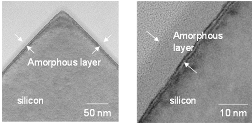
図Ⅲ-2-(二)-B-16 テクスチャ表面へリンイオンを注入したときに形成されたアモルファス層
