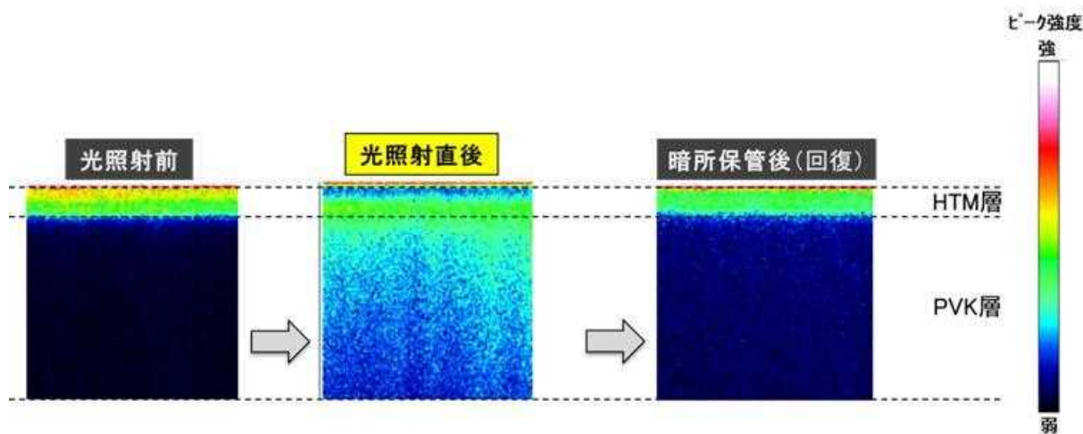
図III-2-(ハ)-D-11 Sym-HTPcH-5 に Li 系添加剤を用いたペロブスカイトセルの照射前後のホール輸送層/ペロブスカイト層界面近傍の Li の分布状態の変化(SIMS) (セル構成：TCO/c-TiO 2 /m-TiO 2 /MAPbI 3 /Sym-HTPcH-5/Au)
