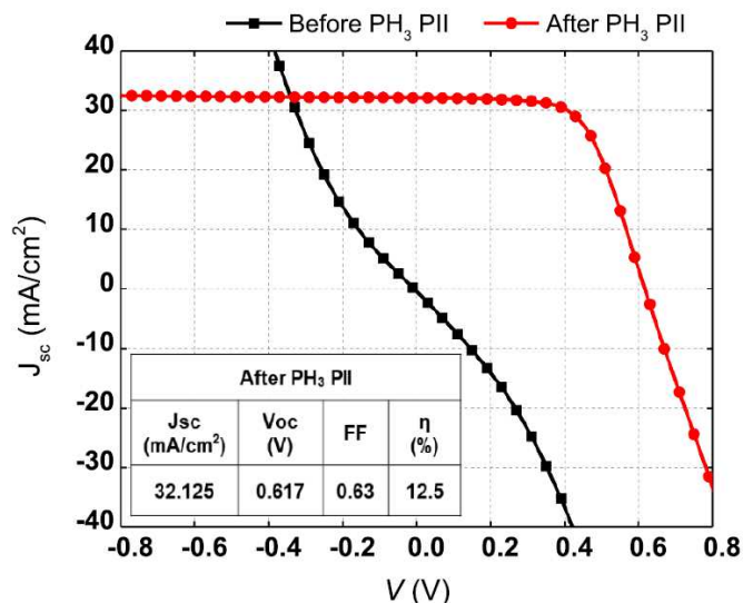
図III-2-(ニ)-C-12 p-a-Si への \text{PH}_3 イオン注入で形成した n-a-Si を有する SHJ 太陽電池の J - V 特性
