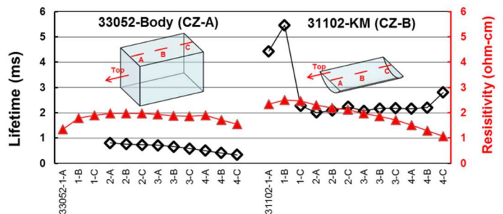
図Ⅲ-2-(二)-A-3 従来手法(CZ-A)と改良手法(CZ-B)によって成長したインゴットのライフタイム(黒)と抵抗率(赤)の分布
