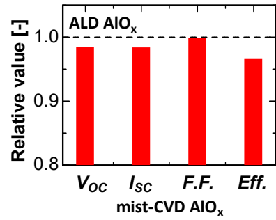
図Ⅲ-2-(二)-A-45 ミストCVD法による \text{AlO}_x 膜を導入した PERC セルと ALD 法による \text{AlO}_x 膜を導入した PERC セルとの相対比較
