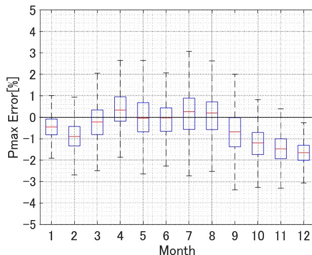
図V-2 PVストリングにおける測定・評価結果
