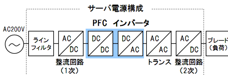
図Ⅱ.1.2.1-2 サーバ電源の構成ブロック図
