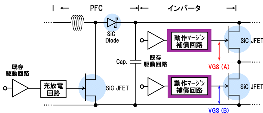
図Ⅲ.2.1.2.2-5 動作マージン補償回路
