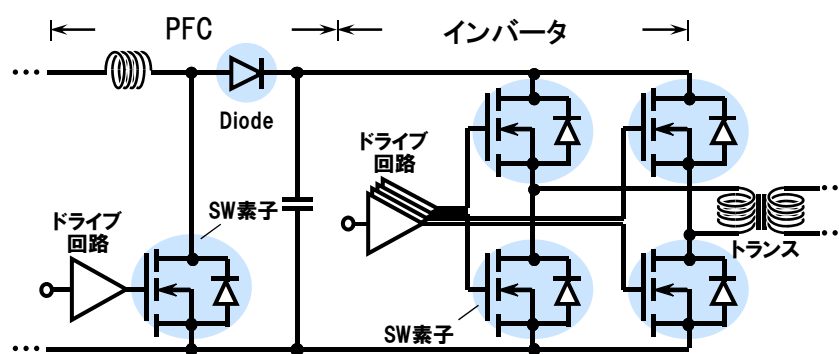
図Ⅱ.1.2.1-3 サーバ電源の構成回路図
