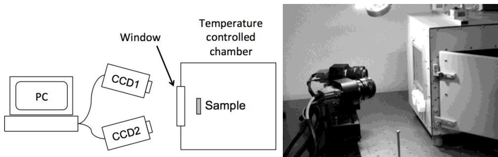
図III.2.3.2.4-4 熱変形評価装置のセットアップ
