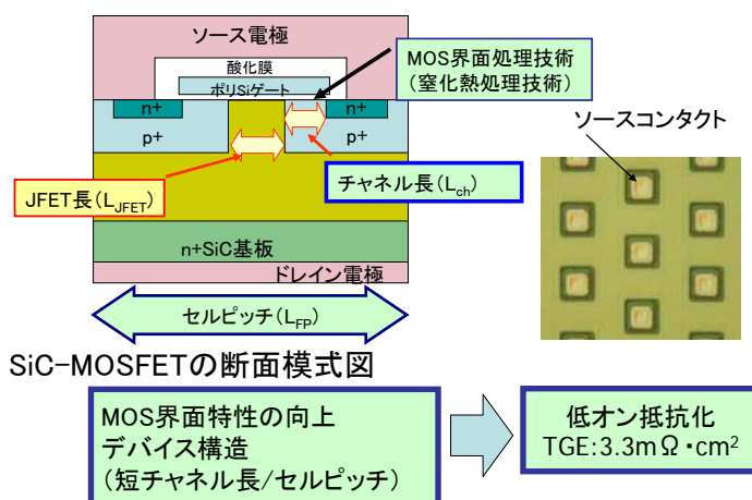
図 III.2.2.1.1-1 SiC-MOSFET の断面模式図
