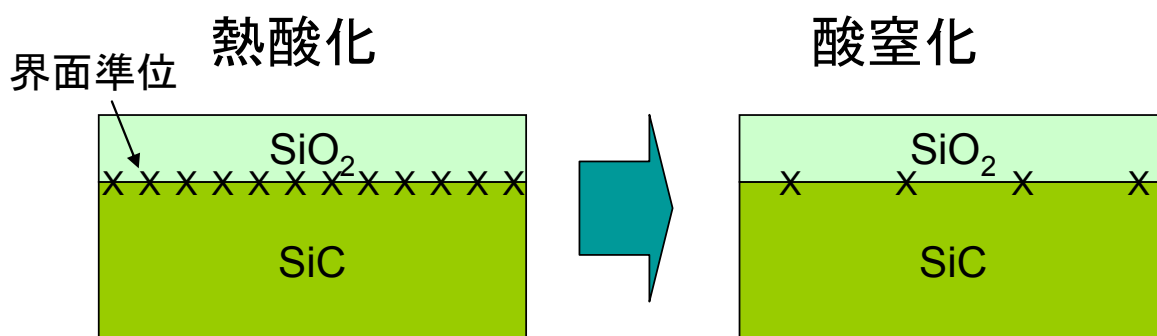
図Ⅲ.2.2.1.1-2 ゲート形成方法
