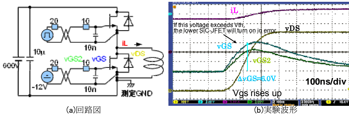
図III.2.3.2-13 SiC パワーデバイスのダブルパルス試験
