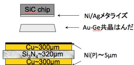
図 III.2.3.2.3-5 SiC チップ / AMC 配線基板の断面模式図
