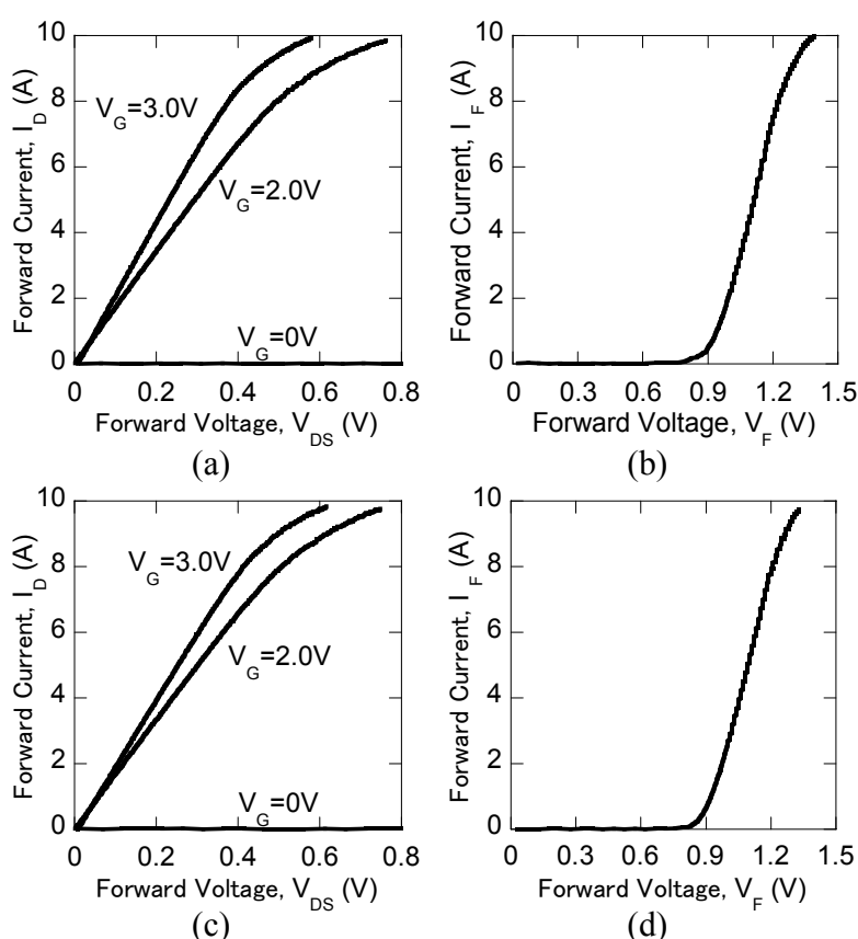
図 III.2.3.2.3-18 作製した両面モジュールに組み込まれている SiC-JFET のドレイン電流 ( I_D )-ドレイン電圧 ( V_{DS} ) 特性のゲート電圧 ( V_G ) 依存性、及び、SiC-SBD の順方向特性。(a)(b) モジュール作製直後、(c)(d)- 40^{\circ}\text{C} ~ 250^{\circ}\text{C} 冷熱サイクル 500 回後。
