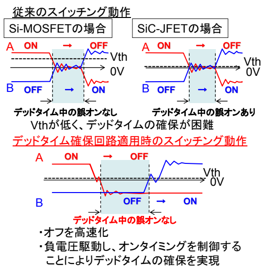
図Ⅲ.2.1.2.2-6 動作マージン補償回路の動作原理
