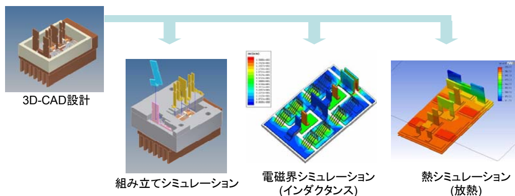
図III.2.3.2.2-21 3D-CAD を利用した CAE 解析結果
