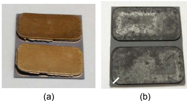
図Ⅲ.2.3.2.1-16 -40°C⇄250°C冷熱サイクル試験に掛けたSiN基板の外観: (a) Cu-SiN (100サイクル後) and (b) CIC-SiN (1万サイクル後)
