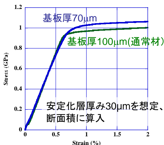
図 2.4.4-6 厚みの異なる基板を用いて PLD により成膜した線材の応力-歪み曲線
