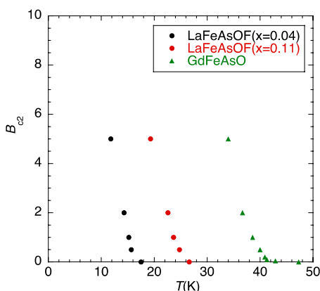
図 2.4.2-98 \text{LaFeAsO}_{1-x}\text{F}_x ( x = 0.04, 0.11 ) と \text{GdFeAsO}_{1-x} 単結晶の B_{c2} の温度依存性。
