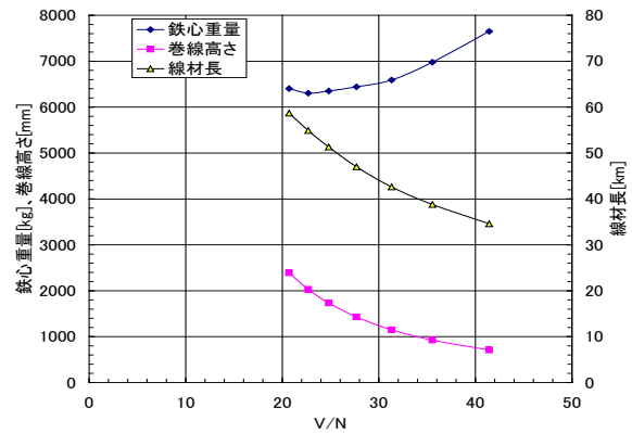
図 2.3.5-37 鉄心重量、巻線高さ及び線材長の V/N 依存性
