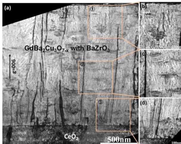
図 2.4.2-40 (a) BZO ナノロッド添加長尺 GdBCO 線材の断面 TEM 写真。(b)-(d) は (a) の領域①-③の拡大写真
