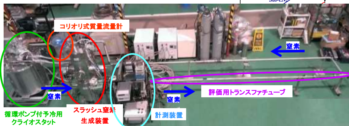
図 2.2.6-16 スラッシュ窒素循環試験装置写真
