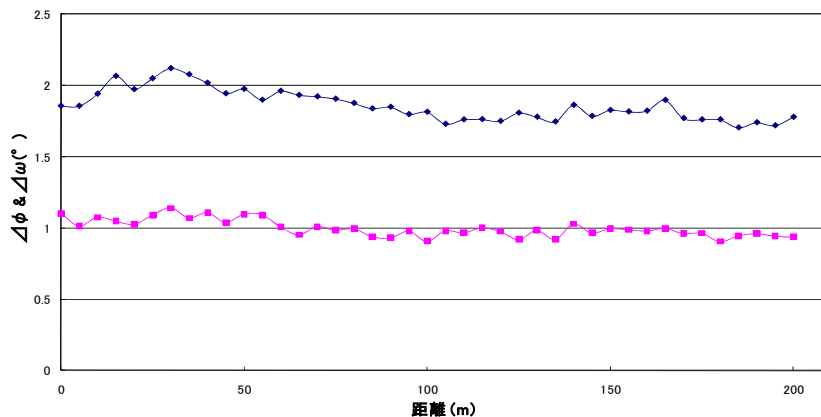
図 2.4.3-2 PLD-CeO 2 /スパッタ-LMO/IBAD-MgO/スパッタ-GZO/ハステロイ TM 構造の 200 m 長 中間層付き基板の結晶粒の面内配向度の長尺位置依存性
