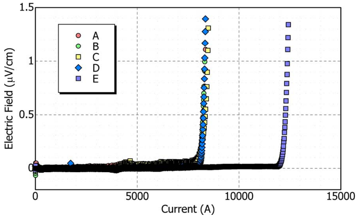
图 2.2.1-28 临界电流测定结果 (@77K)
