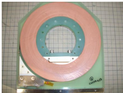
図 2.1.5-2-5 絶縁被覆とパラフィンモールドを施した SP コイルの外観
