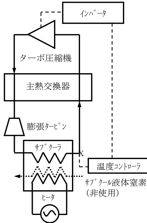
図 2.3.2-33 ネオン冷凍機容量制御フロー
