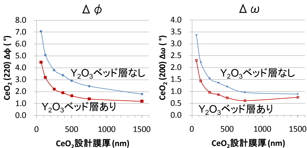
図 2.4.5-3 キャップ層厚みと結晶粒面内 ( \Delta\phi )、面外 ( \Delta\omega ) 配向度の関係における Y 2 O 3 ベッド層挿入の効果
