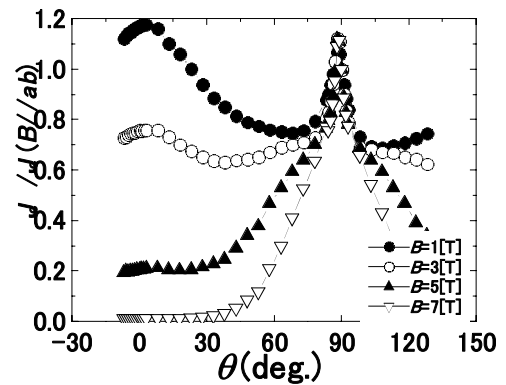
図 2.4.2-11 Y 系超電導線材における規格化 J_c 値の磁場印加角度依存性
