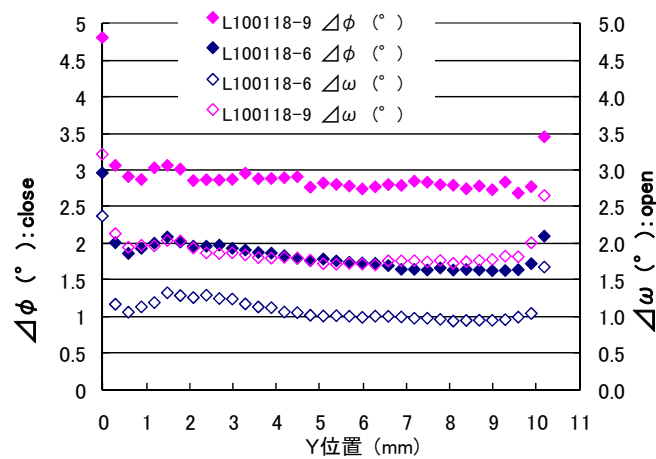
図 2.4.3-1 PLD-CeO 2 /Sputter-LMO/IBAD-MgO/Sputter-GZO/ハステロイ TM 中間層付き基板の結晶粒面内配向度の幅方向分布
