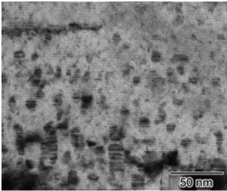
図 2.4.2-38 Zr 添加量 1 mol% 試料の TEM 像
