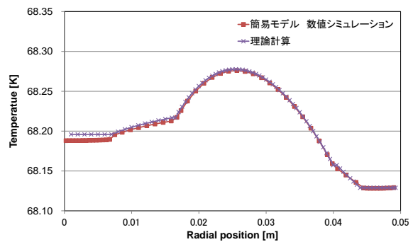
(b) 1000m 地点での半径方向温度分布
