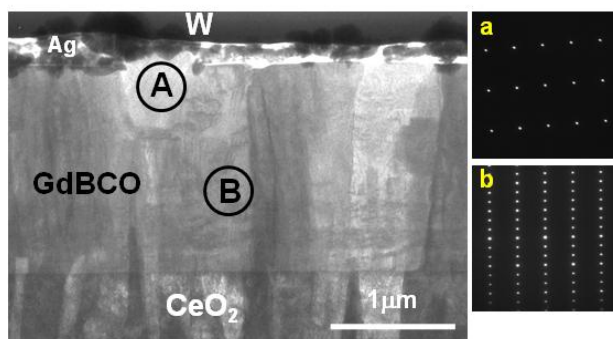
図 2.4.3-66 高 I_c 値領域の PLD-Gd123 層の断面 TEM 像
