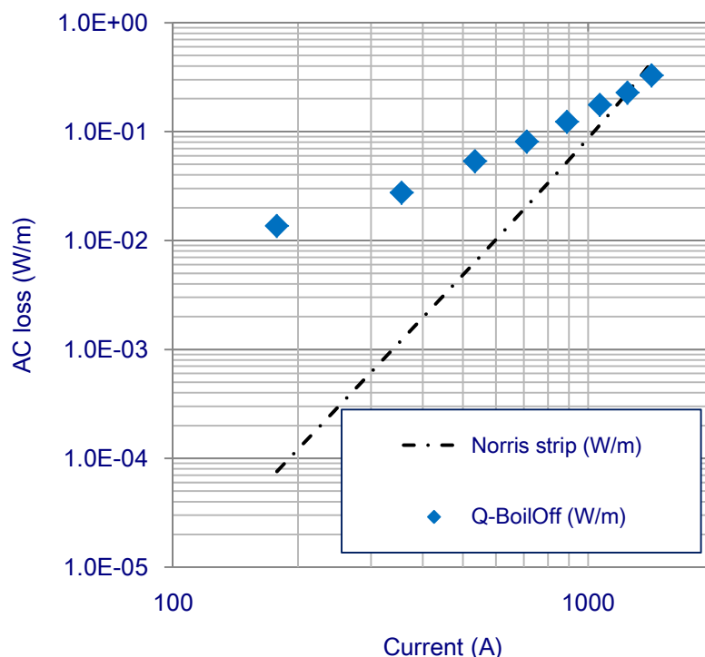
図 2.2.3-38-2 液体窒素蒸発法により測定したシールド層付ケーブルの交流損失
