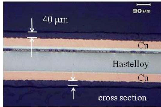
図 2.1.5-2-3 液状樹脂で被覆した超電導線材の断面
