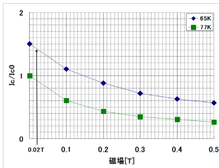
図 2.4.5-63 I_c -B-T 特性
