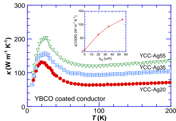
図 2.3.3-26 Y系超電導線材の熱伝導率の温度依存性。挿入図は100 Kにおける伝導率のAg層厚( t_{\text{Ag}} )依存性
