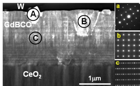
図 2.4.3-67 低 I_c 値領域の PLD-Gd123 層の断面 TEM 像
