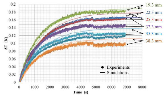
図 2.2.3-50 定常までの温度分布
