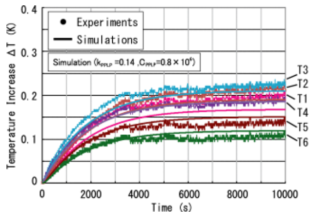
図 2.2.3-45 モデルケーブル A の温度がほぼ定常状態となるまでの時間変化
