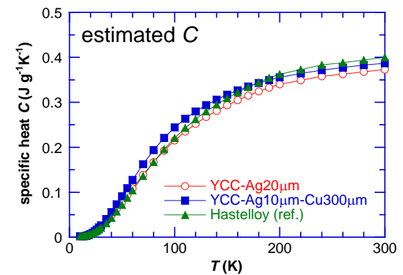
図 2.3.3-34 Y系超電導線材の比熱の推定値
