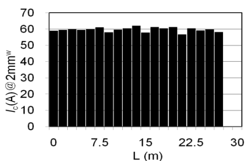
図 2.4.3-49 2 mm-w 線材の I_c 値分布 (30 m 長級)
