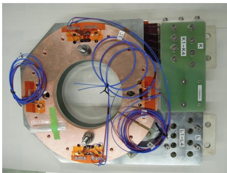
図 2.1.5-4-1 実験に用いた YBCO 集合導体モデルコイル
