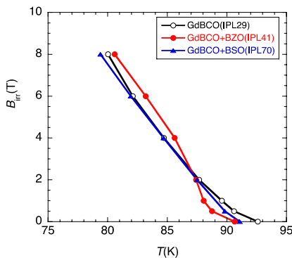
図 2.4.2-85 In-plume PLD 法で成膜した Gd123 における BZO 添加効果
