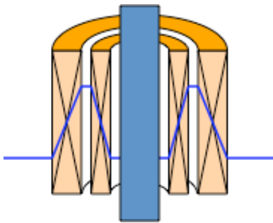
図 2.3.3-17 変圧器巻線における磁界分布
