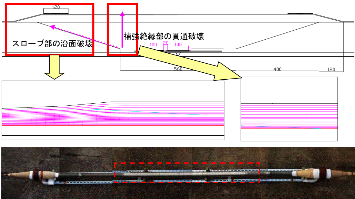
図2.2.3-79 補強絶縁部の破壊用の中間接続部
