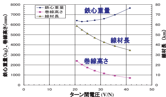
鉄心重量、巻線高さ及び線材長のターン間電圧(V/N)依存性
