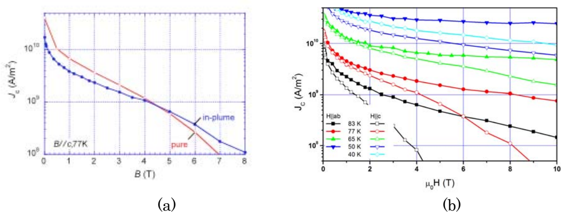
図 2.4.2-84 in-plume 法及び out-of-plume 法による人工ピン無し PLD 線材の磁場中臨界電流特性の比較。(a)77 K、垂直磁場における標準 PLD 試料との比較。(b)広い温度領域を含む垂直磁場、平行磁場中の特性。● : in-plume 法、○ : out-of-plume 法。
