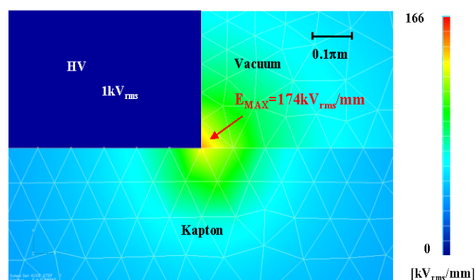
図 2.1.2-4-9 トリプルジャンクション近傍の電界分布
