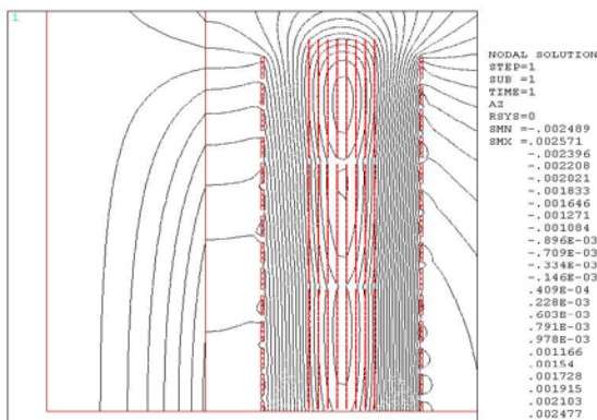
図 2.3.5-41a 磁束線図
