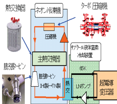
ネオン冷却システムの構成
