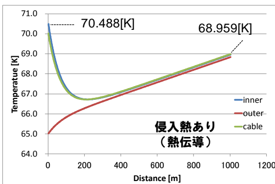
(c) 熱伝導
