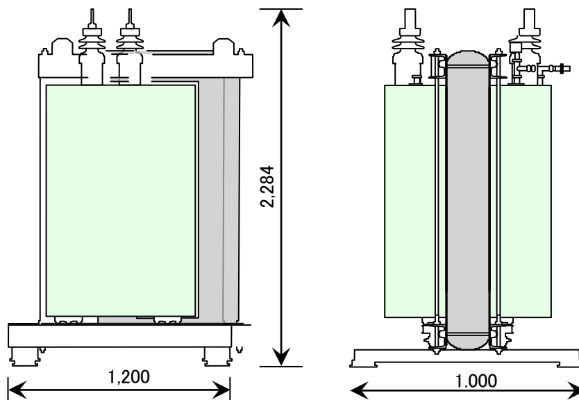
図 2.3.3-42 400 kVA 限流機能付加変圧器モデルの外形
