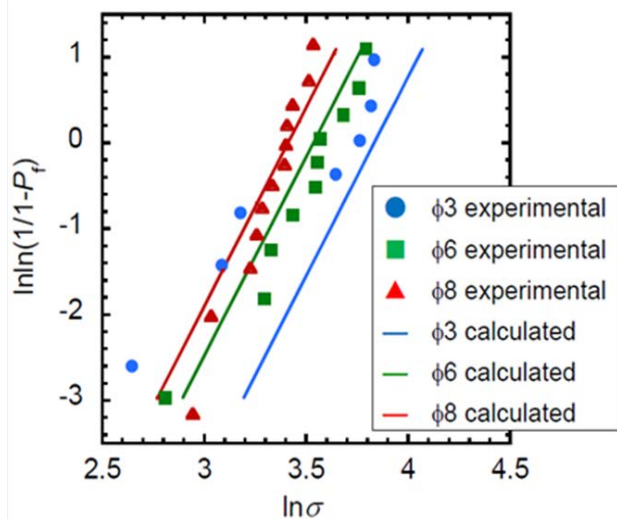
図 2.1.5-1-8 各ロッド径の破壊強度試験結果のワイブルプロット
