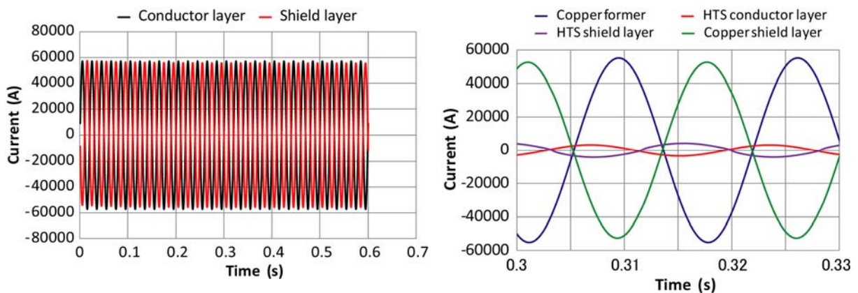
図 2.2.3-58 40 kArms 通電時の電流分布の解析結果
