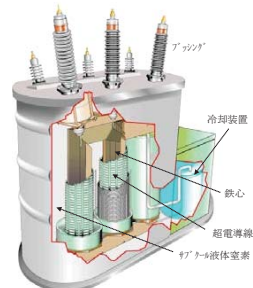
⑤ 20MVA級変圧器 (設計)
