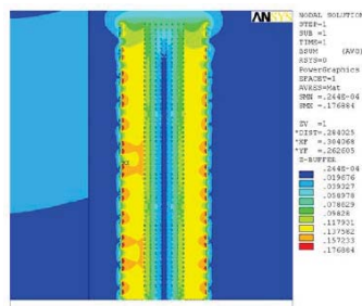
磁界分布
