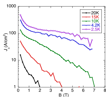
図 2.4.2-99 \text{LaFeAsO}_{1-x}\text{F}_x ( x = 0.11 ) の J_c - B 特性
