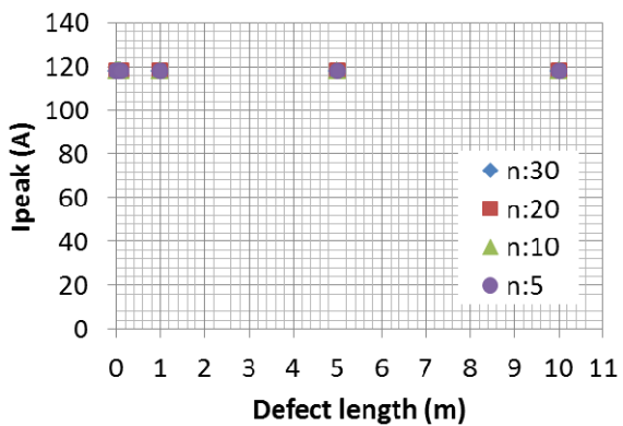
図 2.2.1-73 欠陥素線のピーク電流
