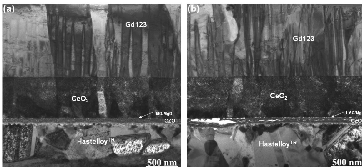
図 2.4.1-39 Gd123/CeO 2 /LaMnO 3 /MgO/MOD-GZO/ハステロイ TM の断面 TEM 像。MOD-GZO 層を(a)600 °Cで焼成、(b)500 °Cで焼成
