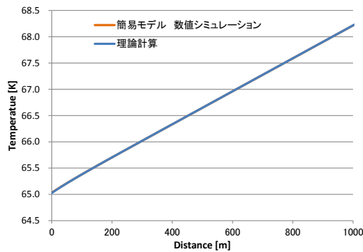
(a) ケーブル長手方向温度分布
