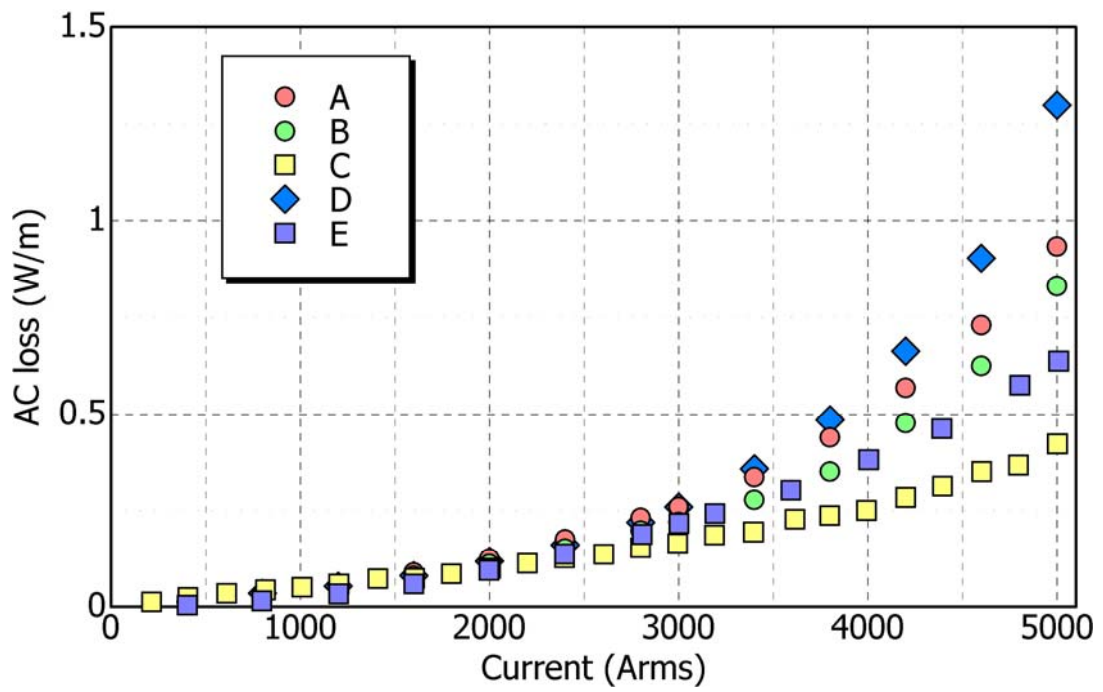
图 2.2.1-29 交流损失测定结果 (@77K)
