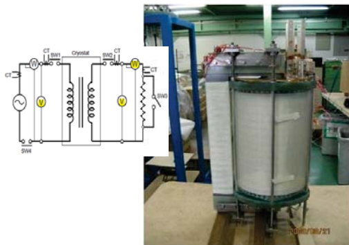
4巻線構造の小型変圧器モデル
