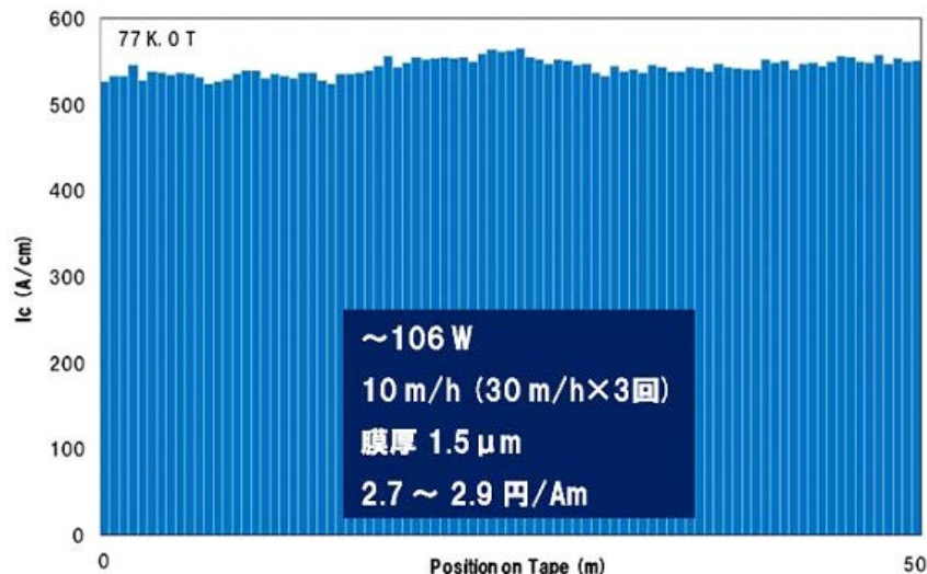
図 2.4.5-12 極低コスト 50 m 長 GdBCO 線材の長手方向 I_c 値分布
