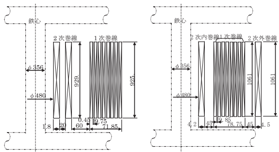
2MVA変圧器の巻線配置 (磁束通路数1) 20MVA変圧器の巻線配置 (磁束通路数2)
