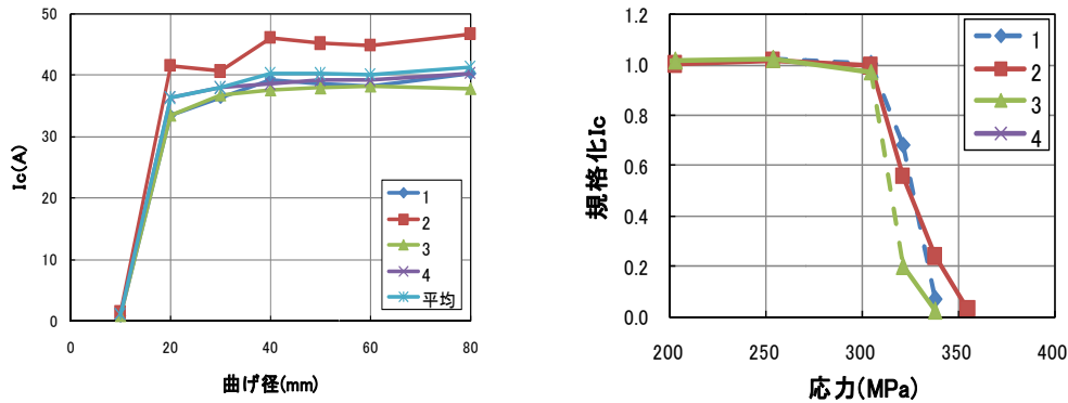
(a) I_c 値の単純曲げ歪み特性
