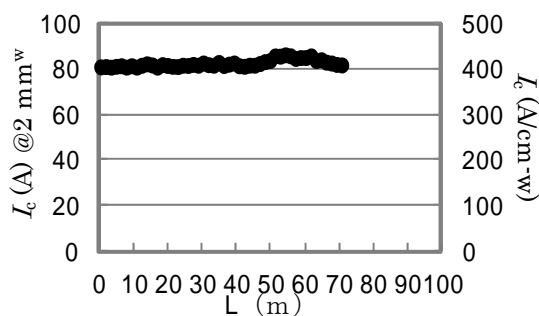
図 2.4.3-50 2 mm-w 線材の I_c 値分布 (70 m 長級)
