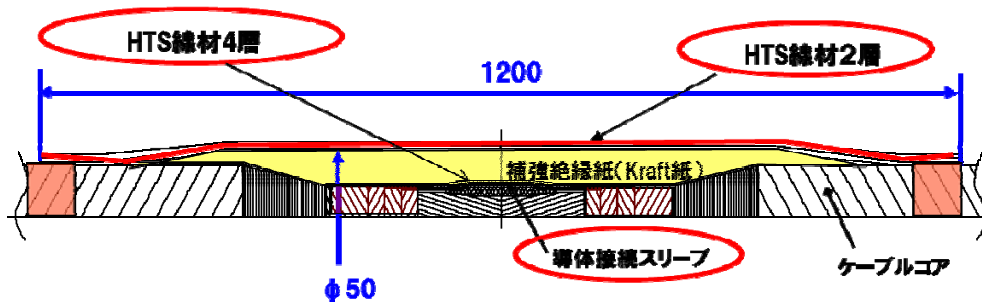
図 2.2.1-91 中間接続部の基本構造
