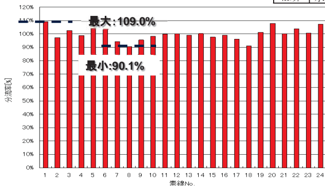
2kA大電流モデルコイルの電流分流率測定結果(66k)
