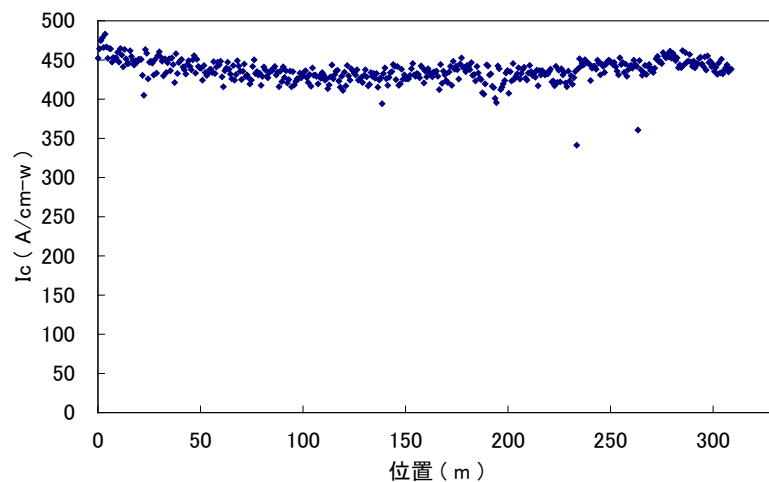
図 2.1.3-2-2 長尺 IBAD-PLD 線材の I_c 値分布図
