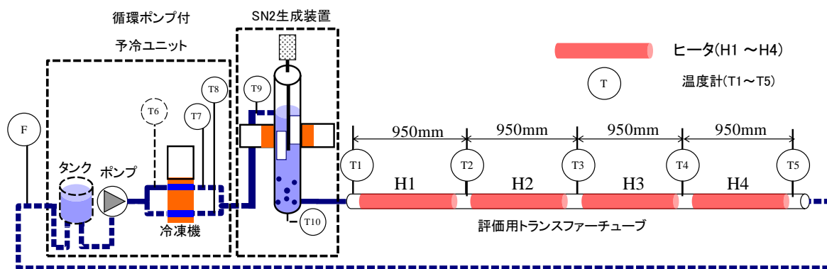
図 2.2.6-15-スラッシュ窒素循環試験装置フロー
