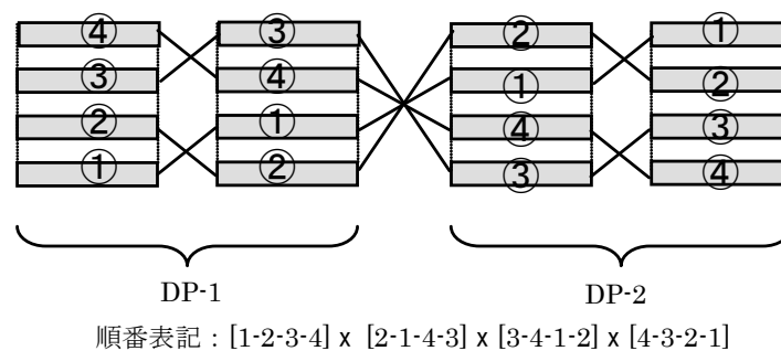
図2.1.1-3-1 1 回の転位のDP配置
