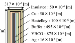
線材の諸元
