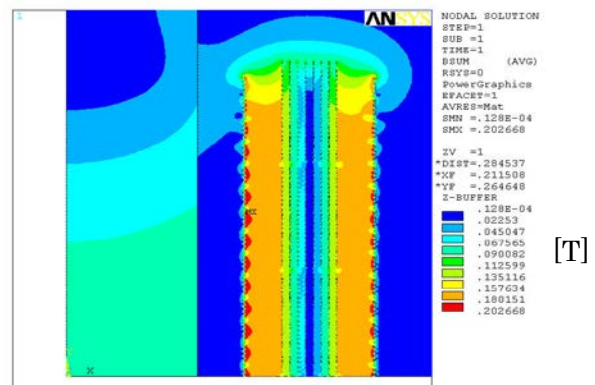
図 2.3.5-41b 磁界分布
