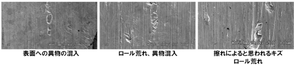
図 2.1.3-1-1 従来基板における表面欠陥の例
