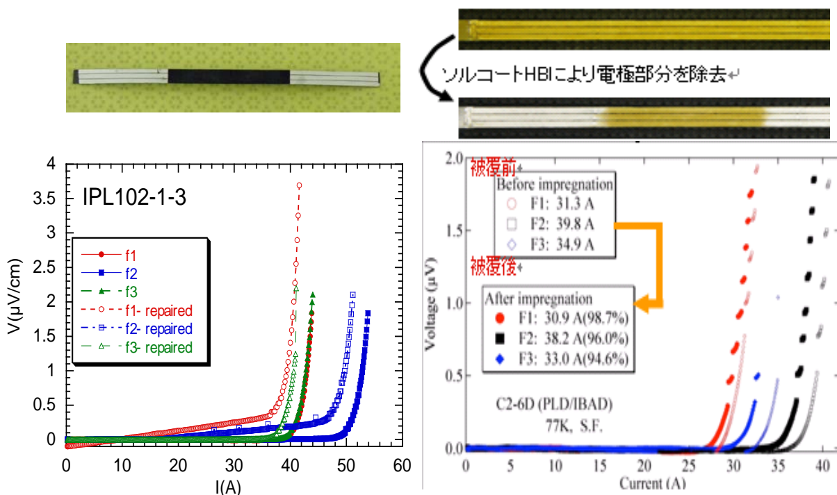
図 2.3.4-36 3分割スクライビング溝加工線材の補修前後の I - V 特性例
