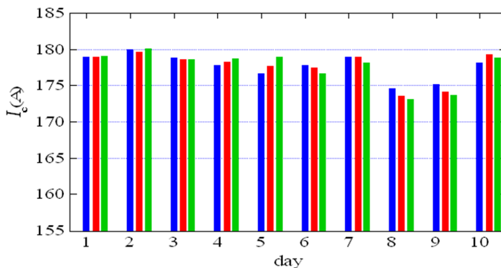
図 2.5.1-3 Lab1 における repeatability と reproducibility を調べるための測定。1 日のうちの 3 回の測定は液体窒素中に浸漬したまま続けて行い、その後室温にて翌日まで保管した。(試料 3-18)
