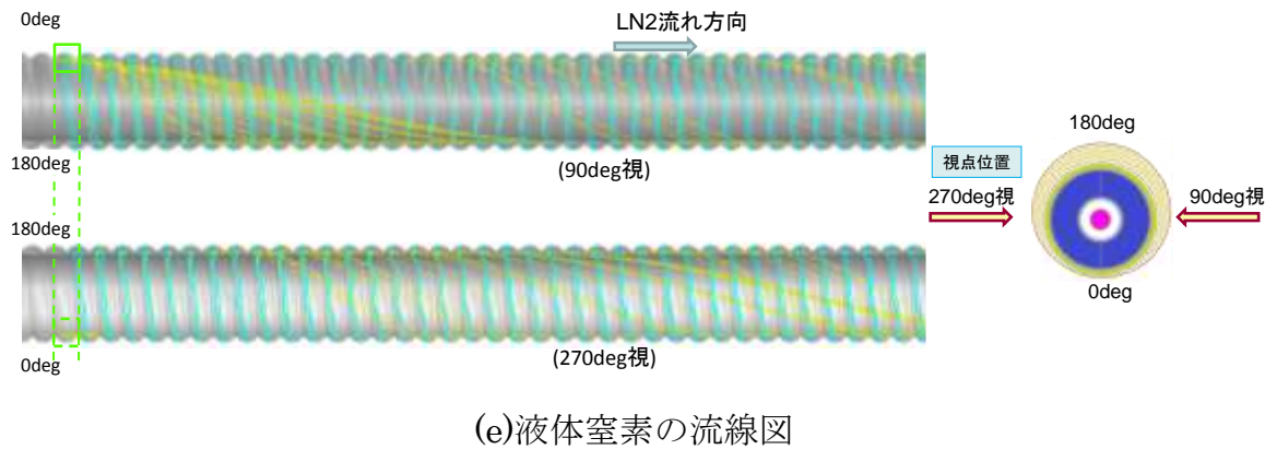
図 2.2.6-26-1 スパイラル・コルゲート管使用時における液体窒素の流体特性 (ケーブル長手方向)
