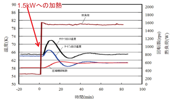
(a)熱負荷ステップアップ 200W→1500W
