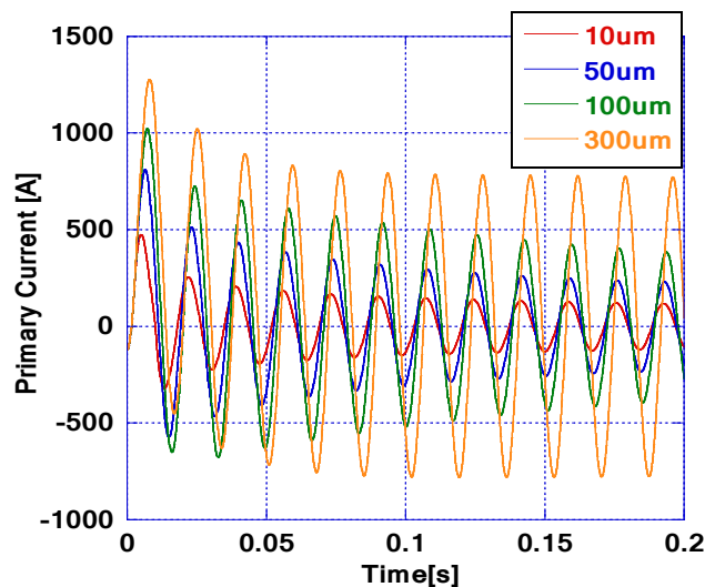
図 2.3.3-21 線材に付加する安定化材の厚さが 10、50、100、300 \mu\text{m} の場合の突発短絡電流の数値解析結果
