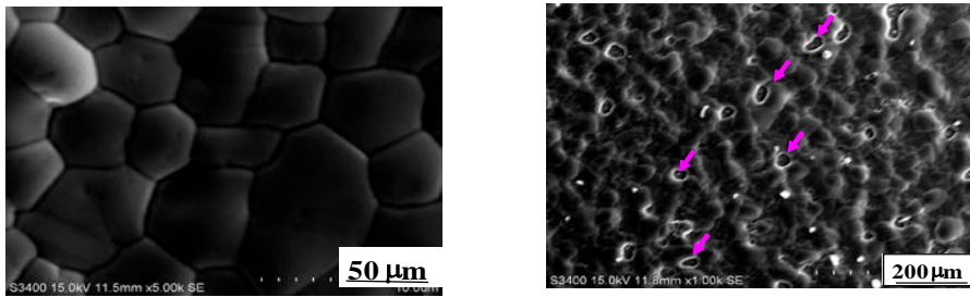
図 2.4.5-56 650°Cで熱処理後 10 \mu\text{m} 厚及び 1 \mu\text{m} 厚の Ag 安定化層の表面形状
