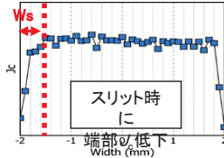
線材幅方向 I_c 分布
