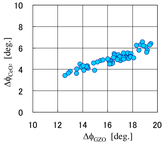
図 2.2.5-21 提供線材の両端から採取した \text{CeO}_2 中間層における結晶粒二軸配向度と IBAD-GZO 層の結晶粒二軸配向度の関係
