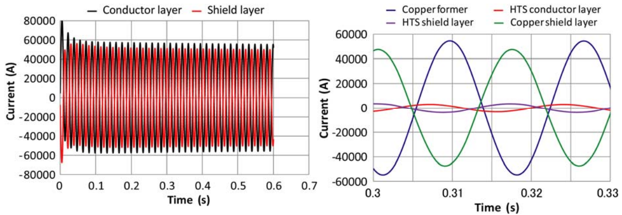
図 2.2.3-57 40 kArms 通電時の電流分布の実験結果
