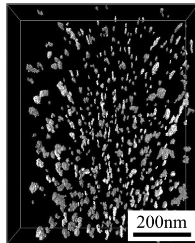
図 2.4.2-48 GdBCO 層内表面近傍における BHO 析出物の三次元再構築像
