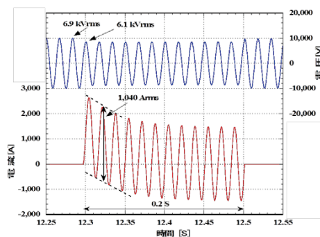
短絡試験時の電圧・電流波形
