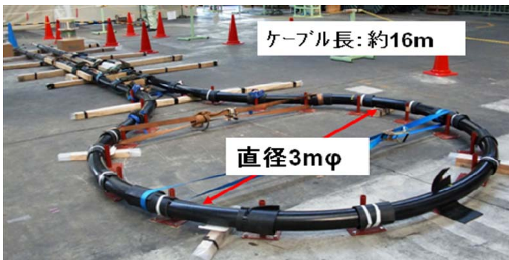
図 2.2.1-40 ケーブル完成後に試験ループに曲げた状態
