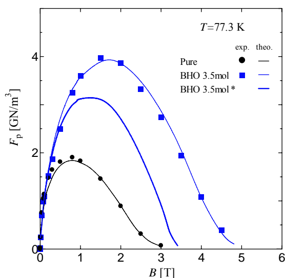
図 2.4.2-55 77.3 K における無添加(●) 及び BHO3.5 mol% 添加試料(■) についての c 軸方向磁場中でのピン止め力密度。中央の太い実線は上部臨界磁場がない場合の特性の理論予想。
