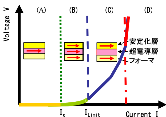
図 2.4.1-2 過電流印加時の電流分流量状態の模式図
