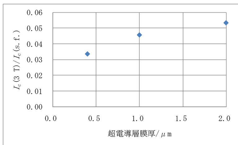
図 2.4.2-1 磁場中 I_c 値の膜厚依存性
