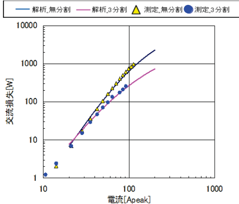
低損失巻線モデルの交流損失測定結果
