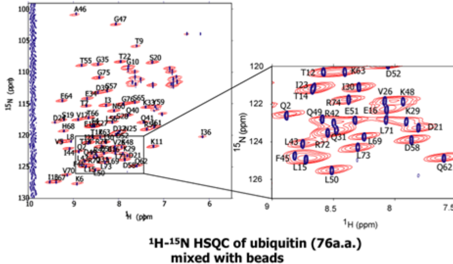
図 35 silica beads 中の Ub の ^1\text{H} - ^{15}\text{N} HSQC スペクトルの重ね合わせ MAS の適用により ^1\text{H} 方向にシグナルが先鋭化し、縮重が解消されたことがわかる。 (赤：非 MAS 条件下 青：MAS 条件下)
