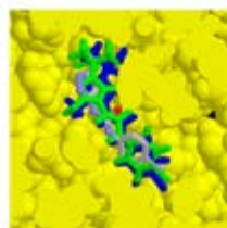
図4 NMR 実験とドッキング計算の融合手法の概念図
