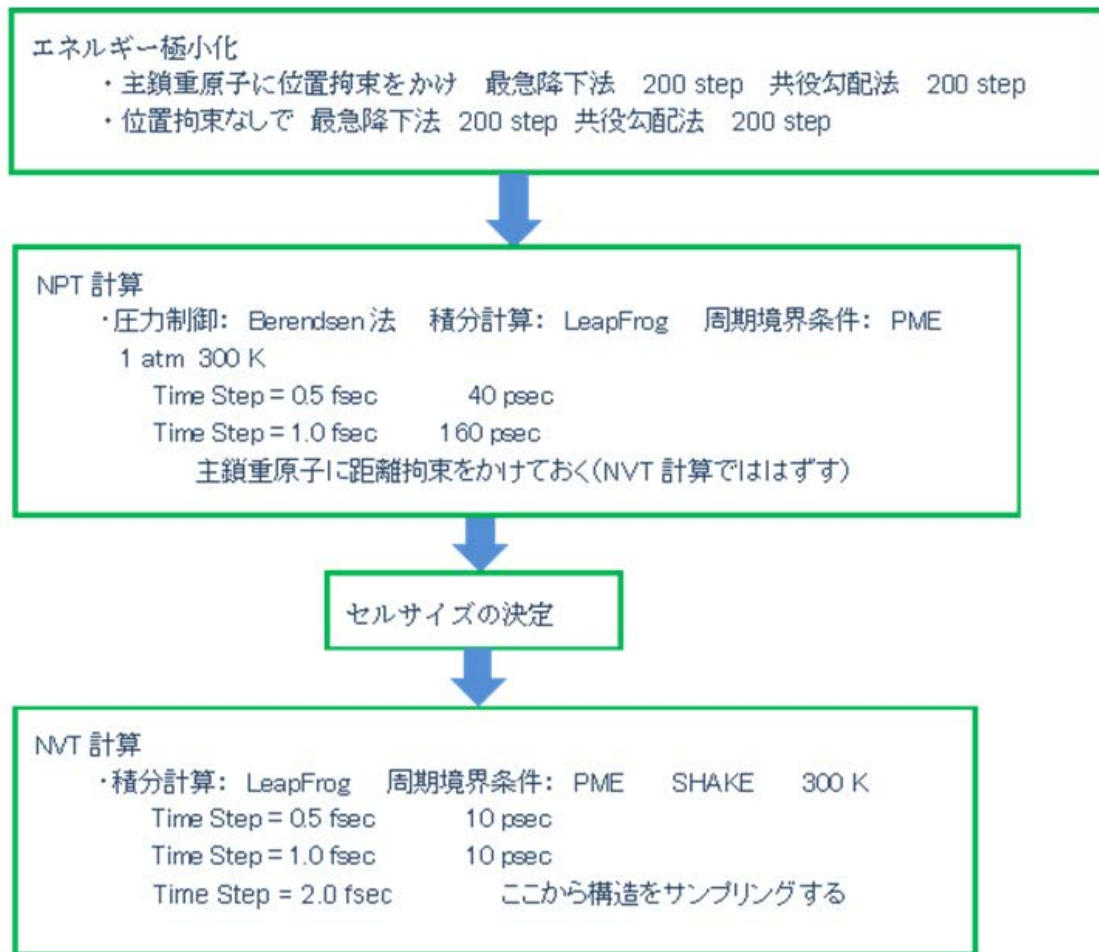
図 43 膜タンパク質のMD計算標準プロトコル
