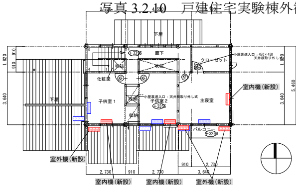
図 3.2.11 戸建住宅実験棟平面図
