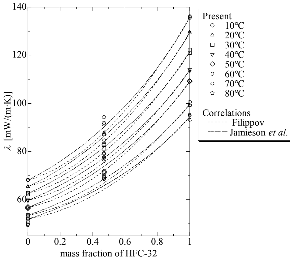
Fig. 5-2 HFO-1234yf+HFC-32 熱伝導率の組成変化
