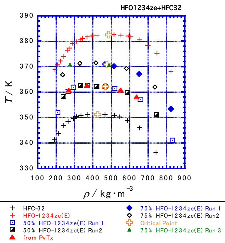
Fig. 1-2-2 HFO-1234ze(E) + HFC-32 系混合物の臨界点近傍における気液共存曲線
