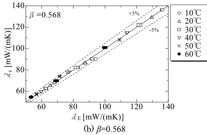
Fig. 5-5 HF0-1234yf+HFC-32 熱伝導率の組成変化の予測結果
