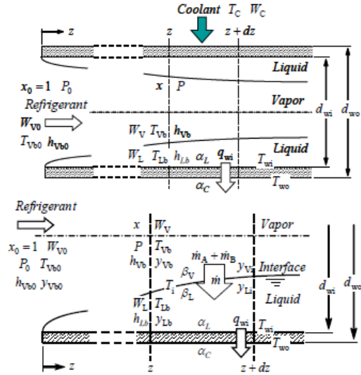
凝縮器熱交換特性予測モデル
