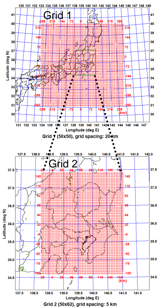
図 4.9：計算対象領域と格子系の子入れ子構造
