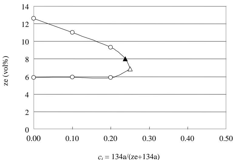
図 2.8 : R-1234ze(E) の燃焼限界に対する R-134a 添加の効果
