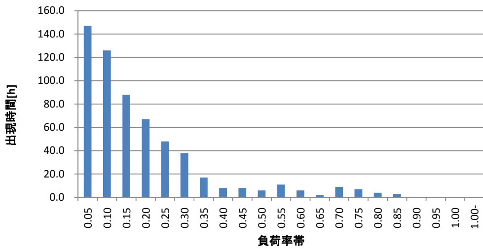
図 3. 2. 47 部分負荷率(冷房、子供室 2)
