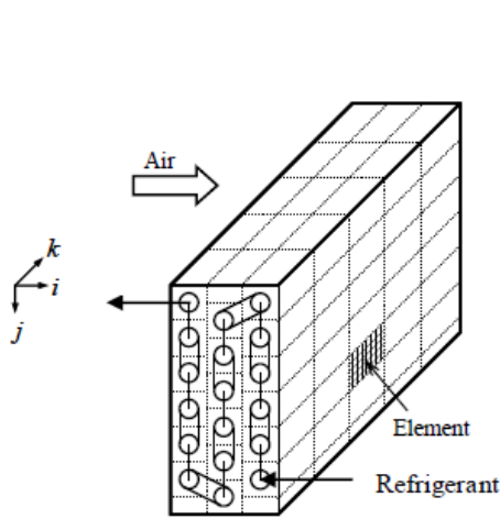
向い直交流型フィン&チューブ式凝縮器
