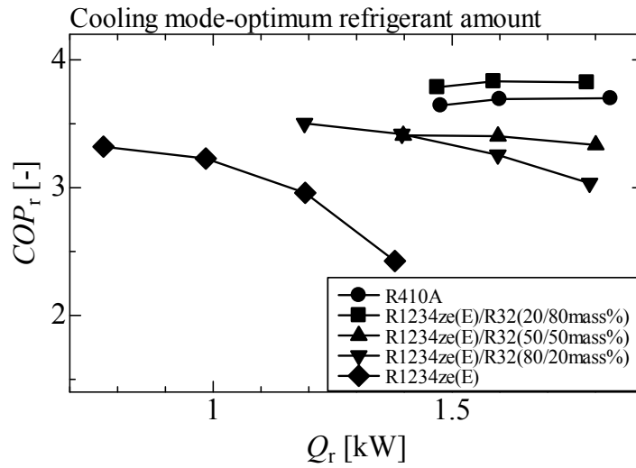
Fig. 4-9 熱交換量による COP_r の変化
