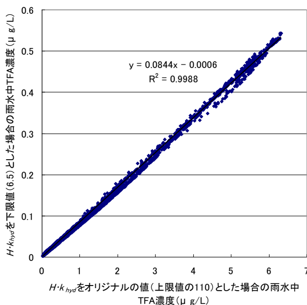
図 4.14 : H \cdot k_{hyd} の実測値の上限値と下限値を使用した場合における雨水中の TFA 雨水濃度の相関関係。TFA 雨水濃度は格子系 2 の大気最下層点で比較した。
