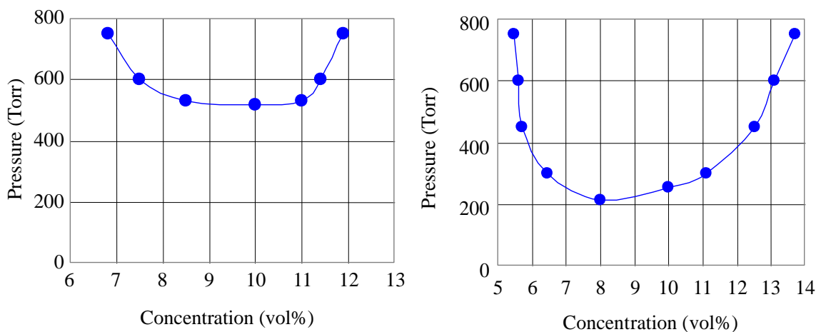
図 2.2 : R-1234yf の燃焼限界に対する減圧効果
