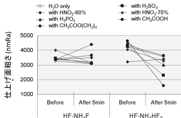
図Ⅲ-2-22 エッチャント組成と仕上げ面粗さ
