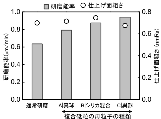
図III-2-4 様々な複合砥粒の研磨特性
