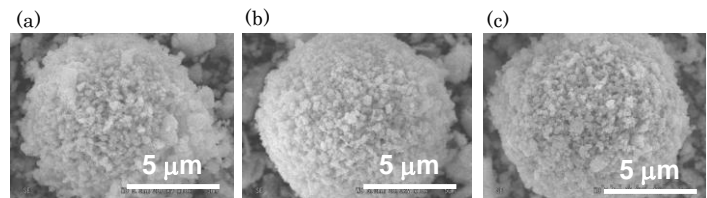
図III-2-3 有機無機複合砥粒のSEM像 (a)真球状粒子、(b)高比重粒子、(c)異形粒子の複合砥粒
