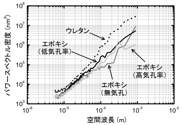
図Ⅲ-2-13 エポキシ樹脂研磨パッドによる研磨後ガラス表面形状の空間周波数解析
