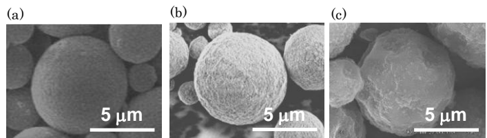
図III-2-2 有機無機複合砥粒の母粒子のSEM像 (a)真球状粒子、(b)高比重粒子、(c)異形粒子
