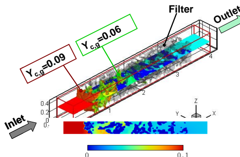
PM濃度の3次元分布計算の一例
