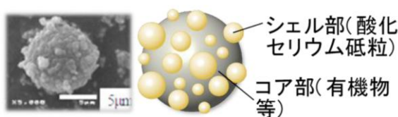
図Ⅲ-1-1 コアシェル構造の有機無機複合砥粒
