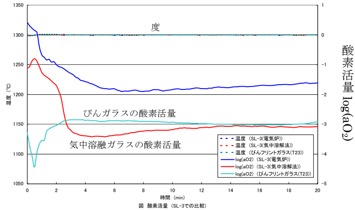
図Ⅲ-2-A3-4. 気中溶解ガラスの溶存酸素量
