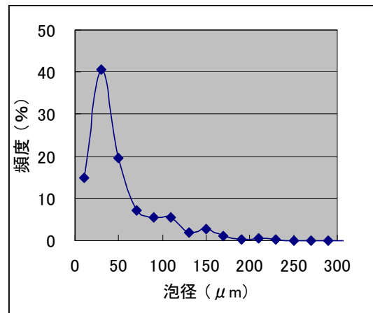
(b) 泡径別の泡数 (38kW, 1530°C)
