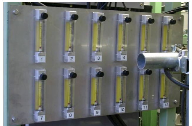
図Ⅲ-2-A1-6. Arガス流量の設定設備
