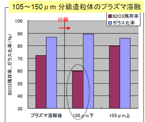
図Ⅲ-2-A2-4. 気中溶融粒子のホウ酸残存率における粒径依存性
