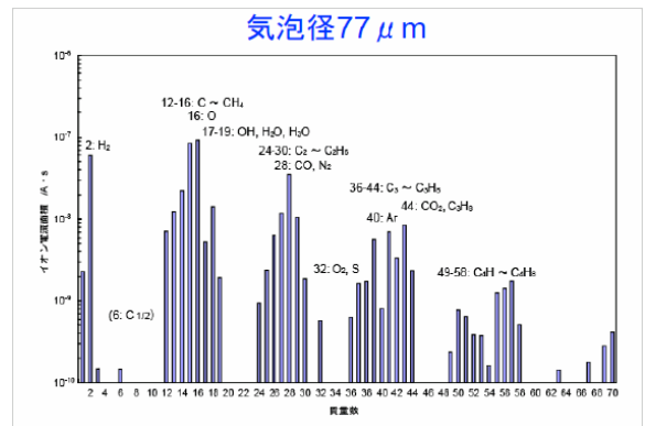
図Ⅲ-2-A5-5. 内包ガスの分析例
