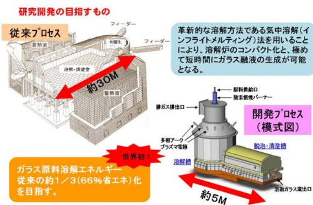
図 I-2-8 従来プロセスと開発プロセスの概略図
