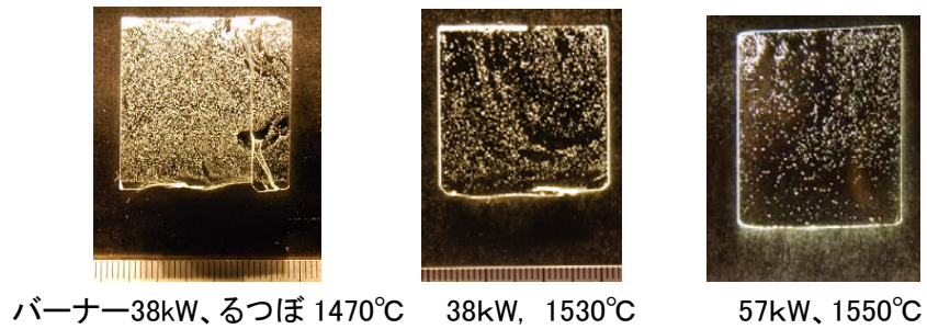
図Ⅲ-2-A2-7. ガラスメルト採取装置の概要と試験状況および採取ガラス例
