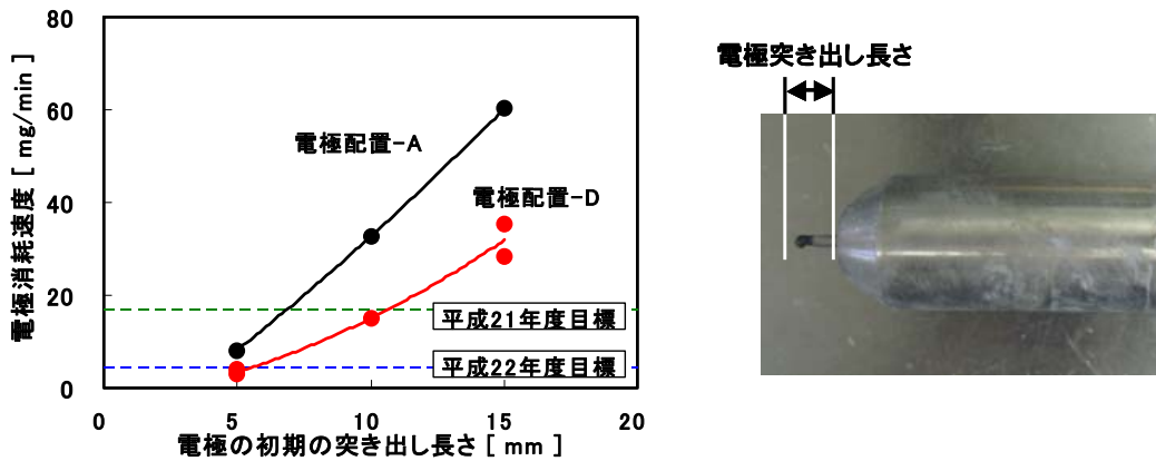
図Ⅲ-2-A1-9. 電極消費速度に及ぼす電極突き出し長さとの電極配置の影響 (電極 1 本当たり 4.17mg/min 以下で 12 本当たり 50mg/min の目標値達成)
