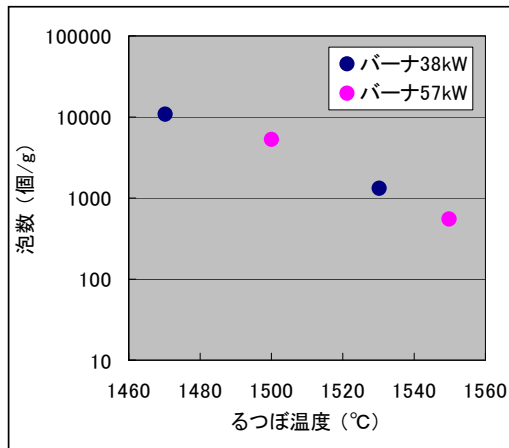
(a) るつぼ温度と泡数
